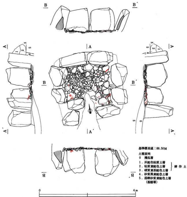
第9圖 龍頭古墳石室實測圖
