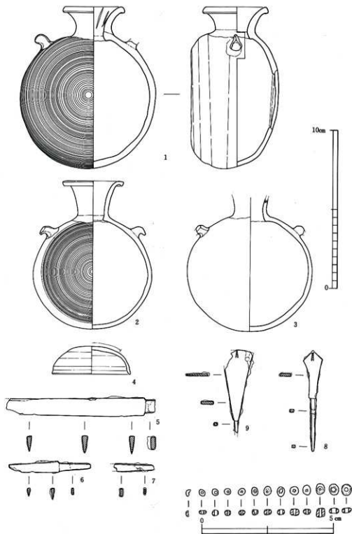
第10图 竜頭古墳出土遺物実測図
