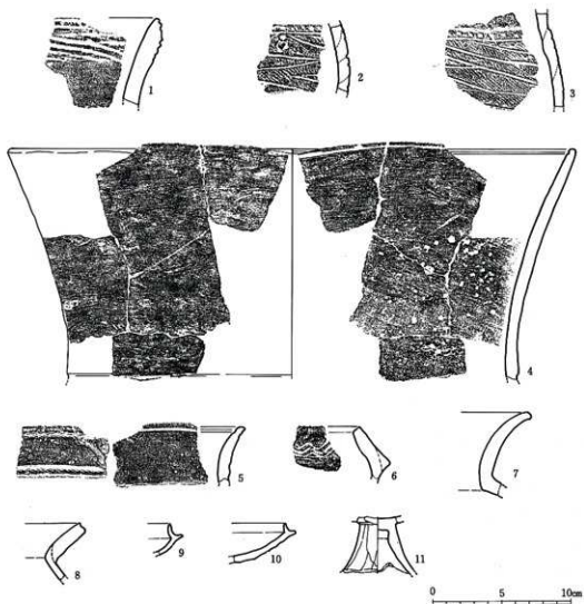
第16図 小田遺跡群出土遺物実例図
