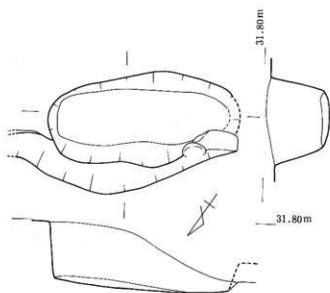
第137图 23号横穴墓前底部1号土坑墓平·断面图
