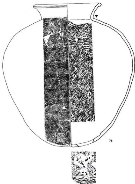
第131图 22号横穴墓出土遺物実測図(4)
