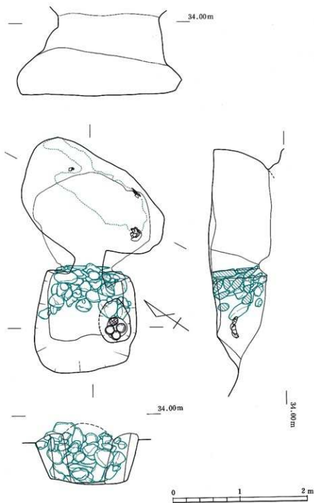
第87图 15号横穴墓平・断面图
