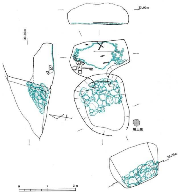
第105图 19号横穴墓平·断面图
