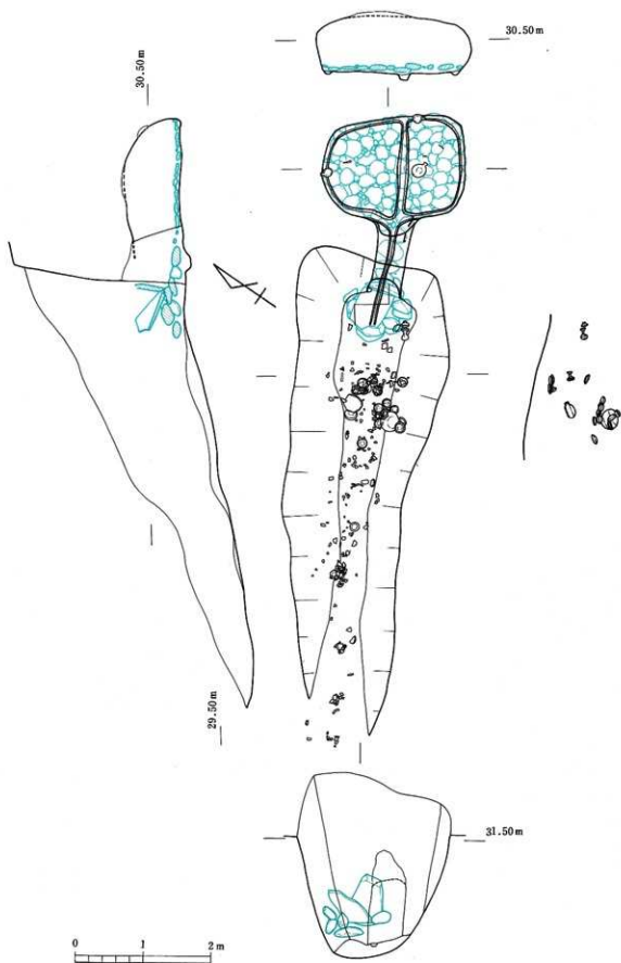
第78图 14号横穴墓平·断面图
