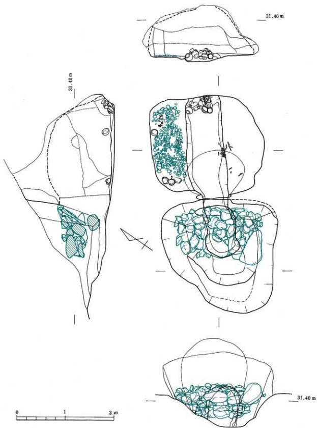
第97图 17号横穴墓平·断面图
