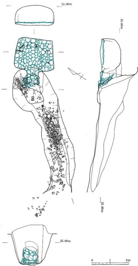
第67图 12号横穴墓平·断面图
