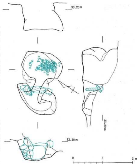
第77図 13号横穴墓平・断面図
