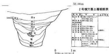
第13図 2号横穴墓横断土層図
