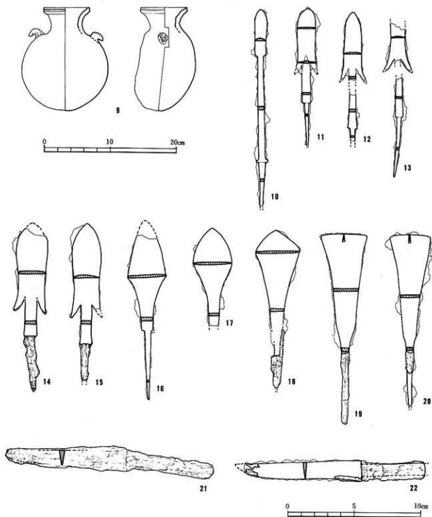
第58図 9号横穴墓出土遺物実測図(2)
