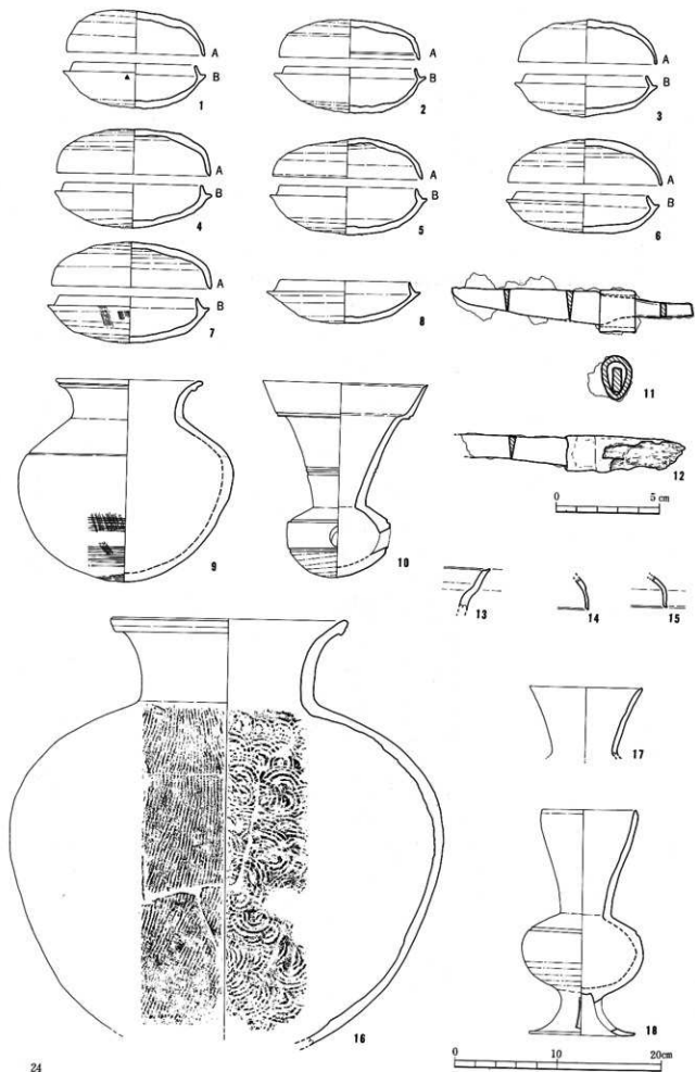
第15图 2号横穴墓出土物实测绘图(1)
