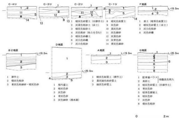
第3図 各トレンチ土層柱状図
