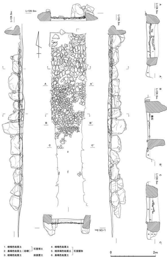
第14圖 圖分61号墳横穴式石室実測圖
