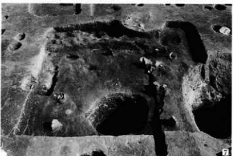
A区18号住居跡
