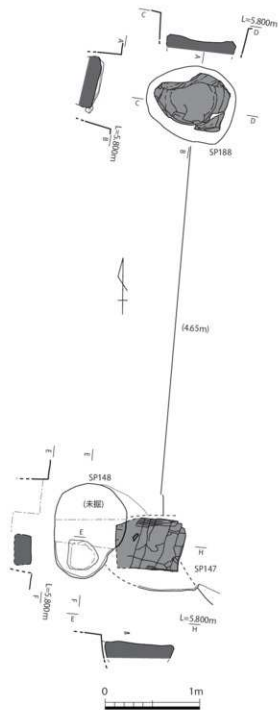
第7-269図 10-SP147・10-SP148・10-SP188実測図(1/40)
