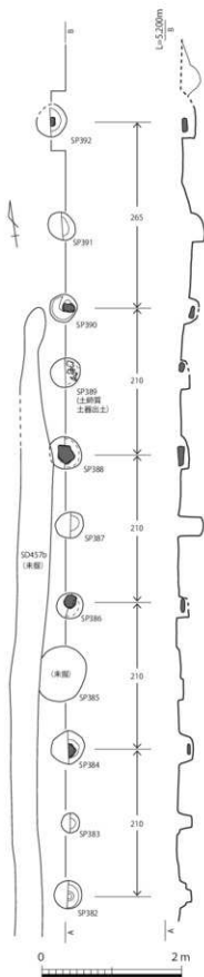
第7-273図 柱穴列実測図 (1/60)
