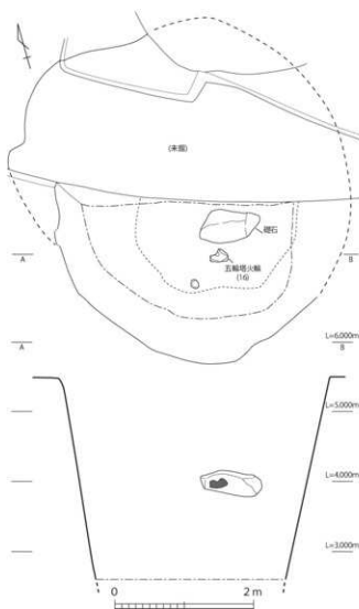
第7-259図 10-SE271実測図(1/50)
