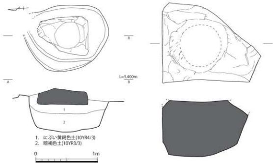
第7-276図 10-SX500実測図 (1/30、1/15)
