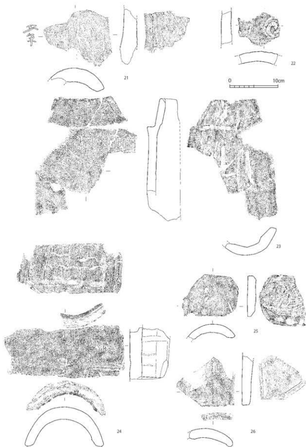
第7-285図 包含層・整地層出土遺物実測図①(1/4)
