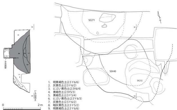
第7-265図 10-SE440実測図 (1/60)
