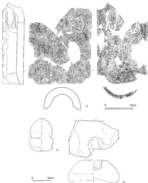
第7-262図 10-SE271出土遺物実測図③ (1/4、1/6)
