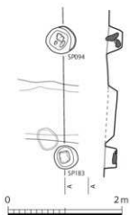
第7-272図 10-SP098ほか実測図 (1/60)
