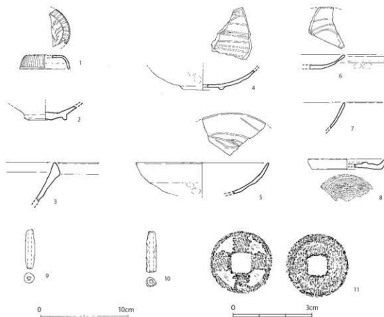
第7-266図 10-SE440出土遺物実測図 (1/3, 1/1)
