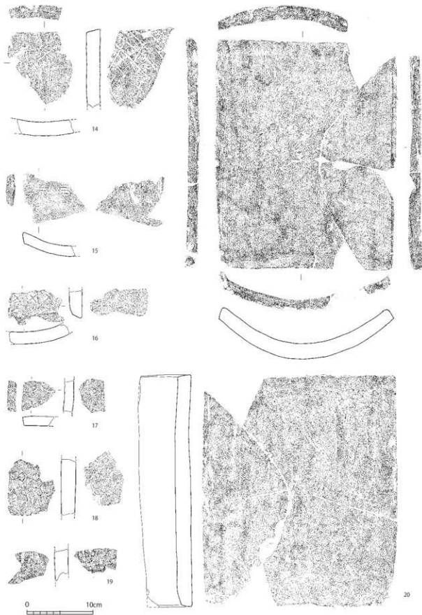
第7-284図 包含層・整地層出土遺物実測図⑧ (1/4)
