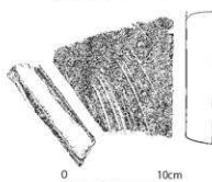
第7-80図 10-SK051出土遺物実測図 (1/3, 1/4)
