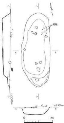
第7-106図 10-SK130実測図 (1/40)
