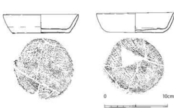
第7-121図 10-SK152出土遺物実測図 (1/3)
