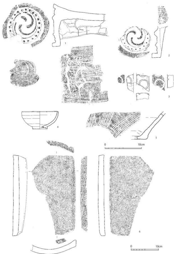
第7-48図 10-SK010a・10-SK010b出土遺物実測図(1/4、1/3)
