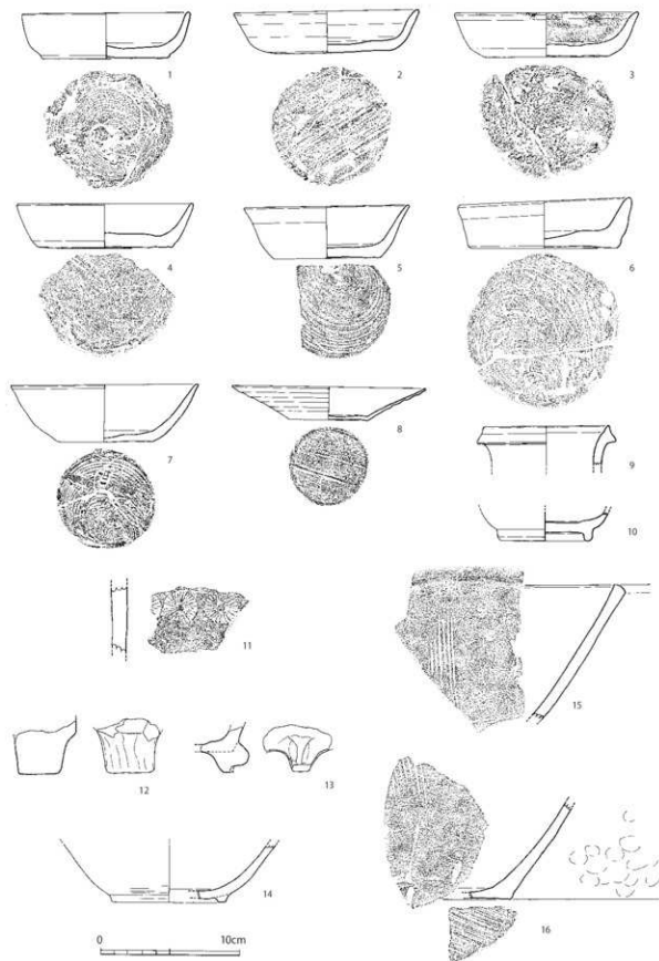
第7-34図 10-SD040出土遺物実測図① (1/3)
