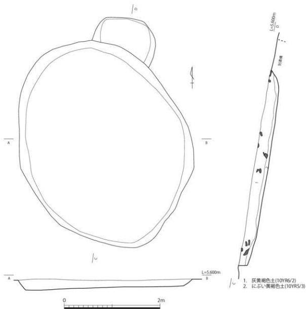
第7-52回 10-SK027実測図 (1/40)
