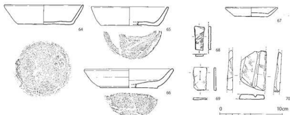
第7-63図 10-SK031出土遺物実測図⑤ (1/3)
