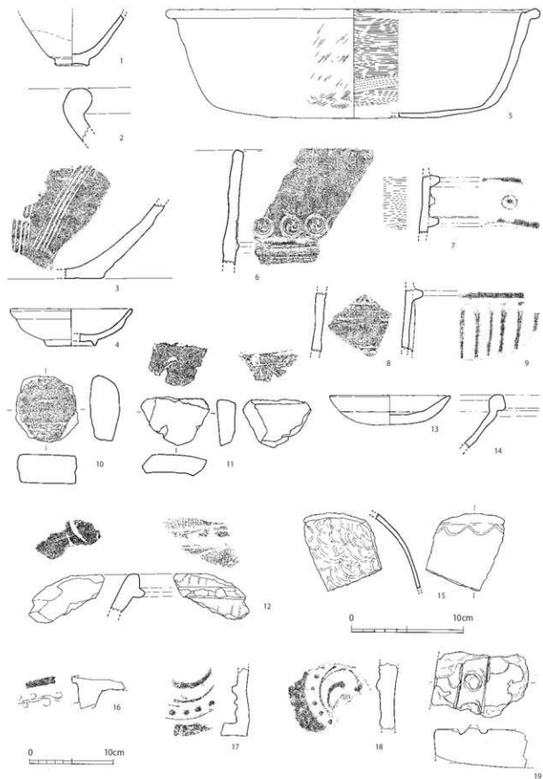
第7-15図 10-SD140出土遺物実測図①(1/3、1/4)
