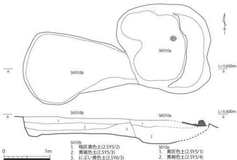
第7-47図 10-SK010a・10-SK010b実測図 (1/40)
