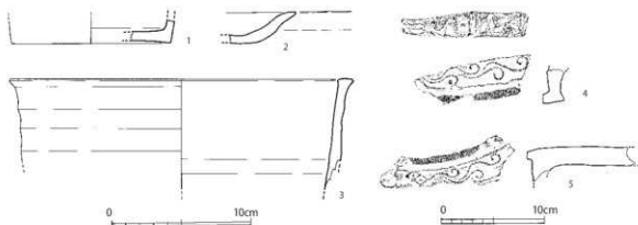
第7-45図 10-SK005出土遺物実測図 (1/3, 1/4)
