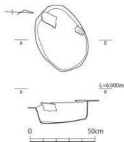
第6-17図 09-SK010実測図 (1/20)
