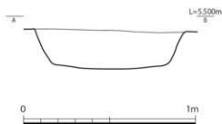
第6-9図 09-SK004実測図 (1/20)
