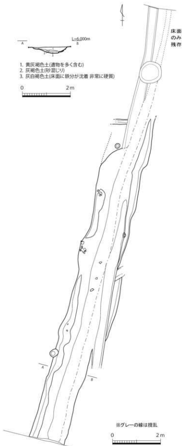
第6-3図 09-SD001実測図 (1/80)
