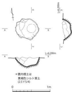
第5-192図 08-SX390実測図 (1/30)
