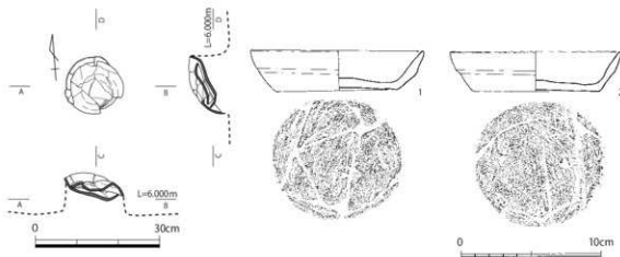
第5-185図 08-SX059実測図(1/10)
