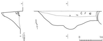
第6-15図 09-SE007実測図 (1/40)
