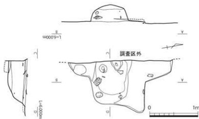
第6-19図 O9-SK013実測図 (1/40)
