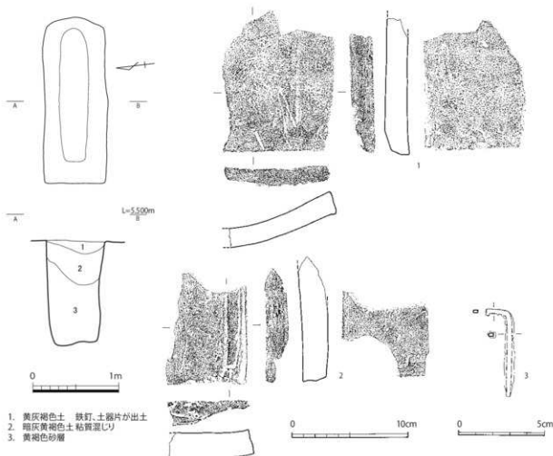
第6-5図 09-SK002実測図(1/40)
