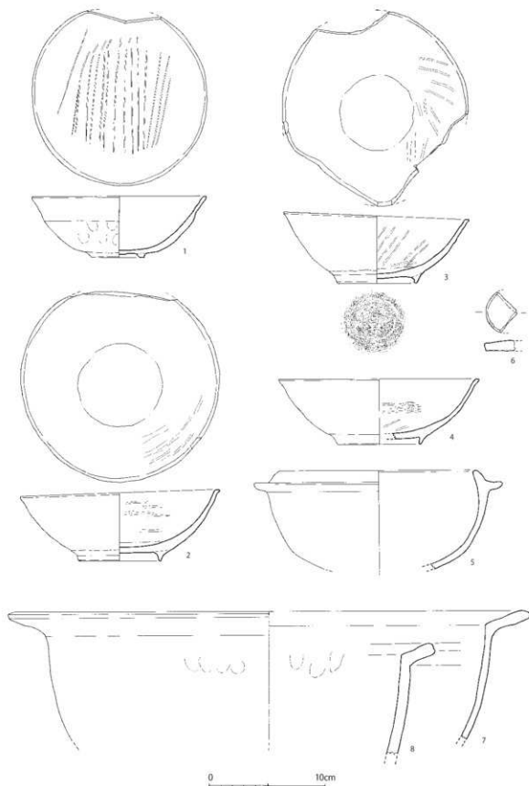
第5-167図 08-SK300出土遺物実測図 (1/3)
