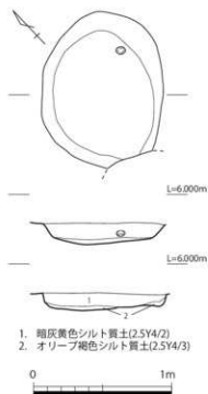
第5-94図 08-SK136実測図 (1/30)
