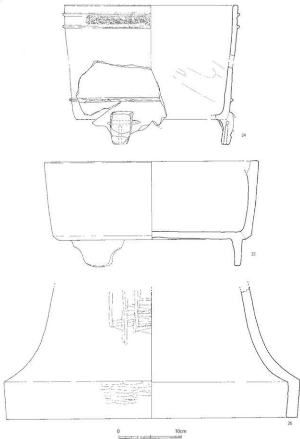
第5-123図 08-SK193a出土遺物実測図⑤ (1/3)
