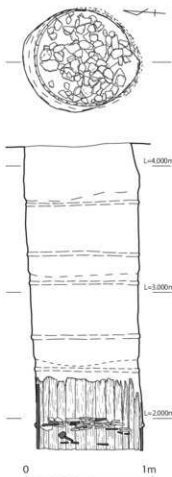
第5-180図 08-SE262実測図② （井筒、1/30）
