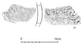
第5-122図 08-SK193a出土遺物実測図④ (1/4, 1/3)
