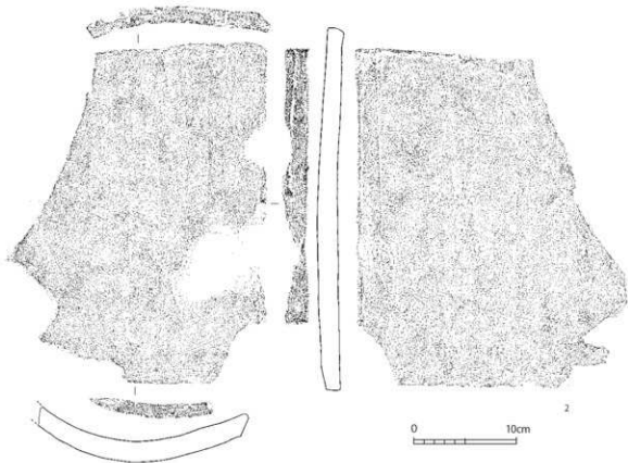
第5-92図 08-SK133出土遺物実測図 (1/3、1/4)
