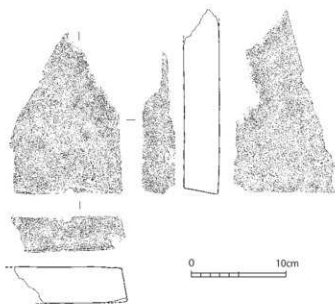
第5-128図 08-SK197出土遺物実測図(1/4)
