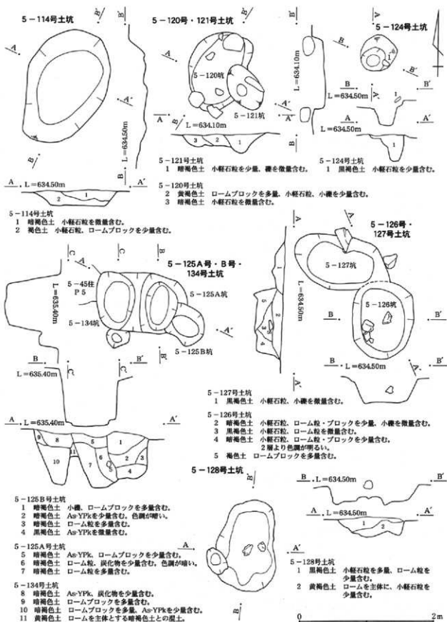
第187図 土坑(20)
