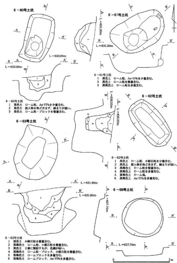
第217図 土坑(50)
