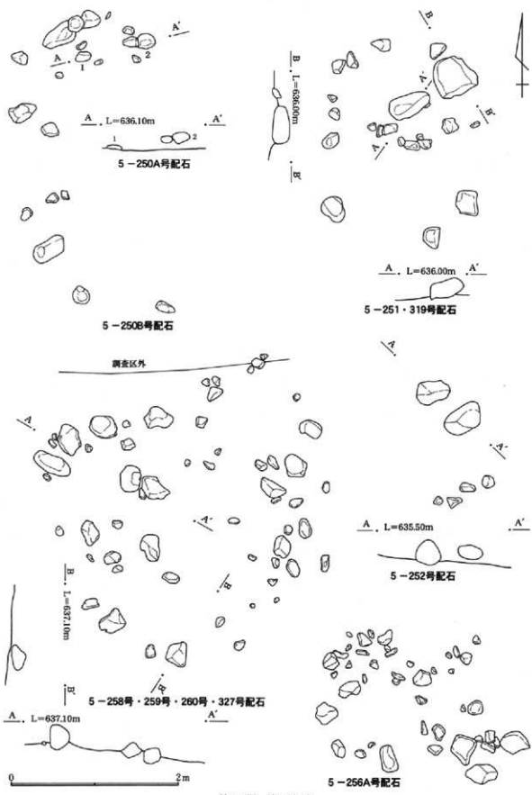
第100図 配石(7)
