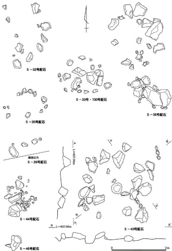
第95図 配石(2)
