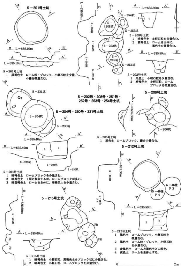
第194図 土坑(27)
