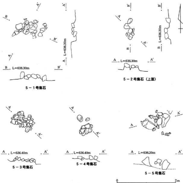
第167图 集石
