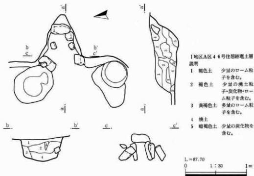
第433図 I地区A区46号住居跡遺構図
