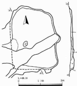
第567図 I地区B区19号住居跡遺構図
