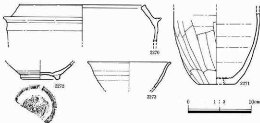
第463図 I地区A区66号住居跡遺物図
