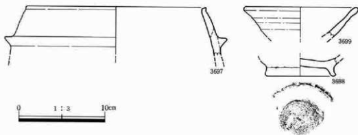
第606図 I地区C区5号住居跡遺物図
