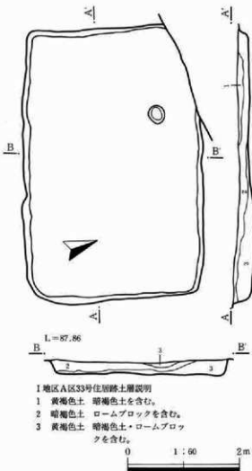
第419図 I 地区 A区33号住居跡遺構図
