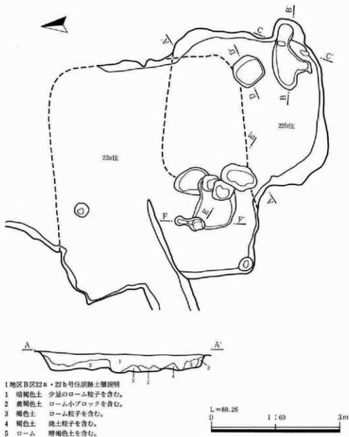
第571図 I地区B区22a・22b号住居跡遺構図(1)
