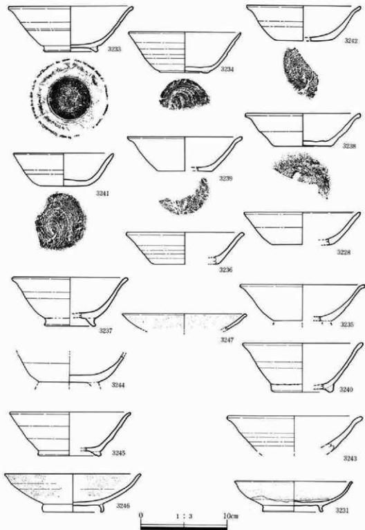
第403图 I地区A区21号住居跡遺物图(3)
