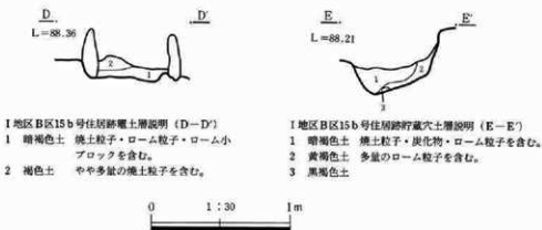
第559図 1地区B区15a・15b住居跡遺構図(2)
