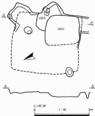
第 457 図 I 地区 A 区 64 号住居跡遺構図
