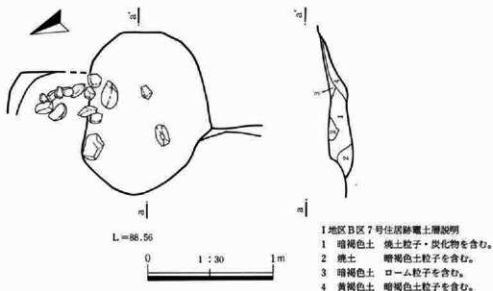
第543図 I地区B区7号住居跡遺構図(2)
