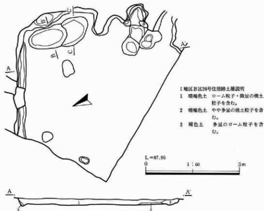
第580図 I地区B区26号住居跡遺構図(1)
