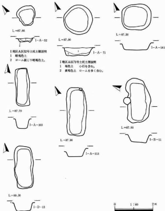
第626図 土坑遺構図
