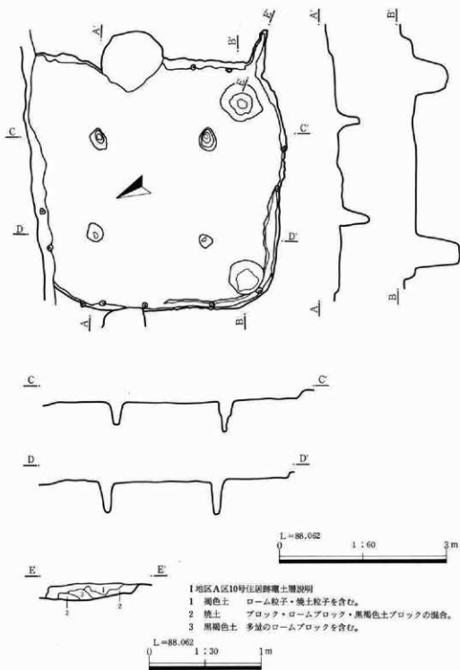
第384図 I 地区A区10号住居跡遺構図
