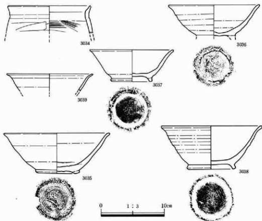
第539図 I地区B区4b号住居跡遺物図
