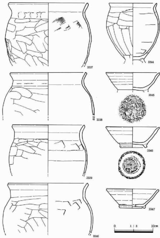
第590图 I地区B区33a号住居跡遺物图(1)
