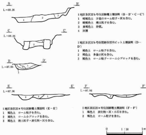
第572図 I地区B区22a・22b号住居跡遺構図(2)
