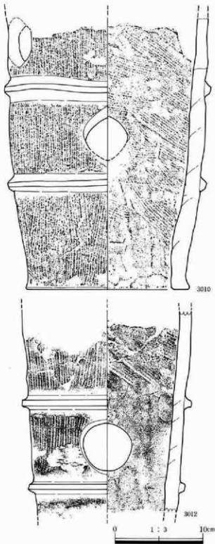
第531図 I地区B区1a号住居跡遺物図(3)
