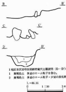
第593図 I地区B区35号住居跡遺構図(2)
