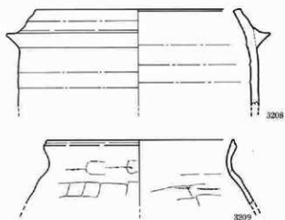
第568図 I地区B区19号住居跡遺物図
