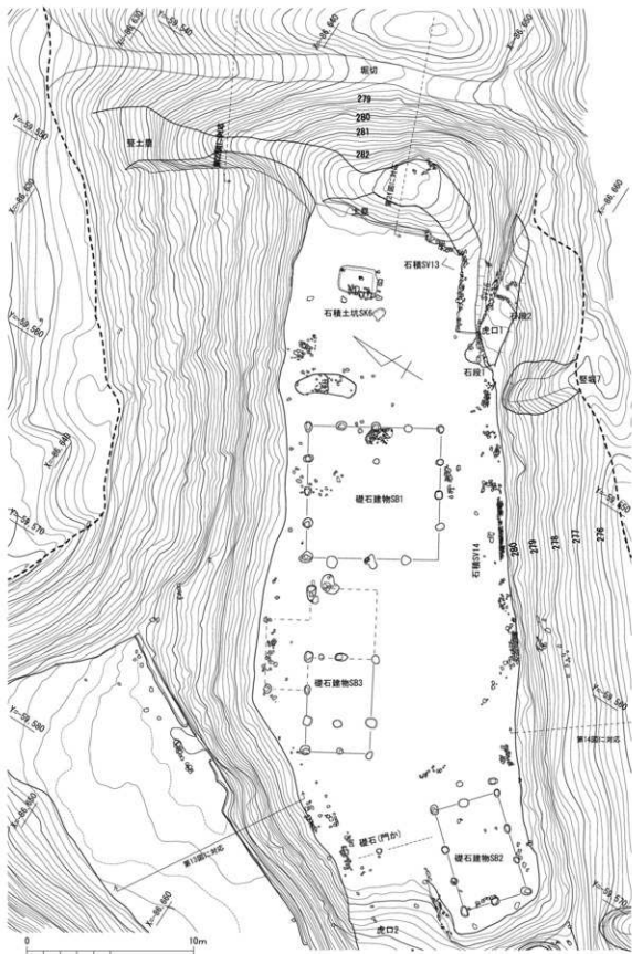
第12図 曲輪1平面図
