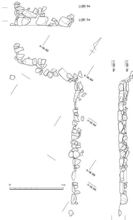
第17図 石積SV13実測図
