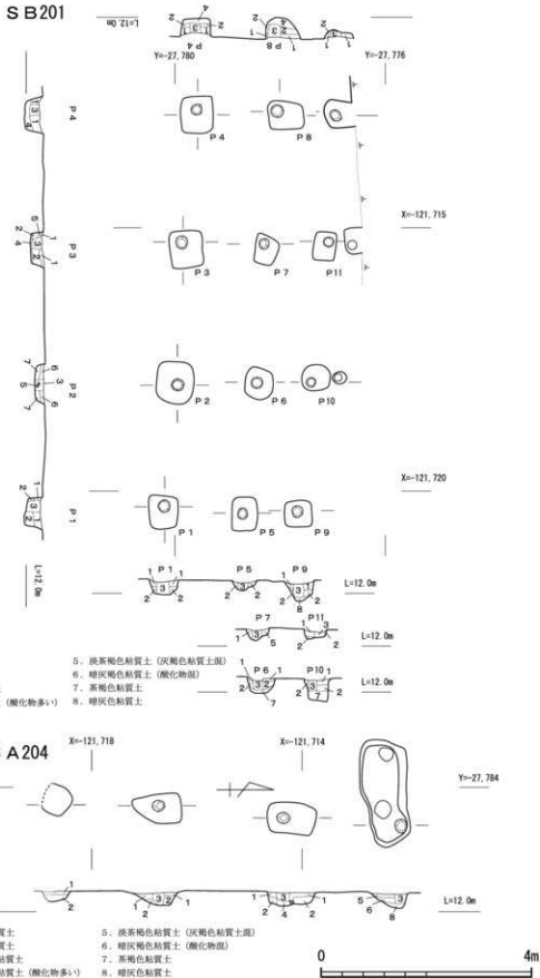
第35図 掘立柱建物跡 S B 201、横列 S A 204実測図
