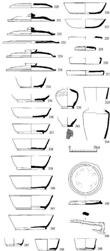
第41図 溝S D 125出土遺物実測図(1)
