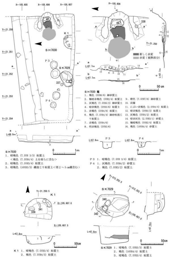
第71図 7区竪穴建物SH7030全体、窟部、土坑平面・断面図
