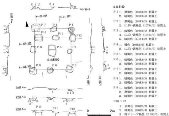
第49図 5区掘立柱建物S B5145・5190平面・断面図
