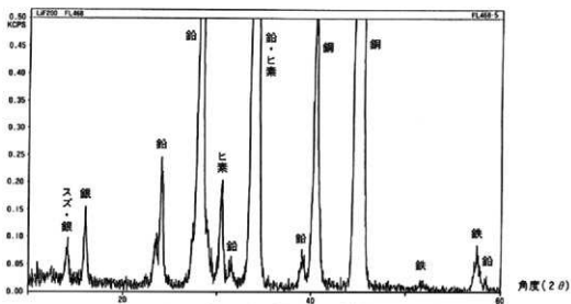
図4-b 図4-aの拡大図
