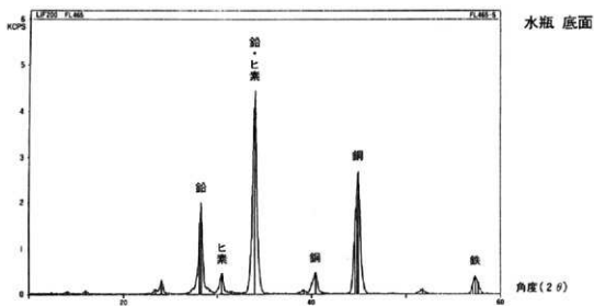
図1-a 和田山天神前遺跡出土水瓶底面の蛍光X線スペクトル図
