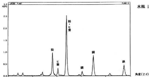
図3-a 和田山天神前遺跡出土水瓶注口の蛍光X線スペクトル図
