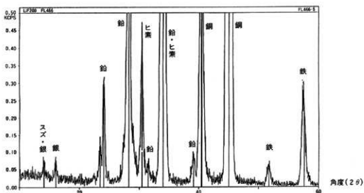
図2-b 図2-aの拡大図
