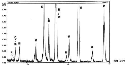
図3-b 図3-aの拡大図
