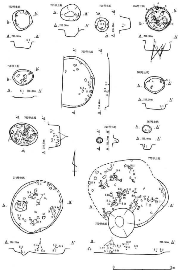
第373図 土坑遺構図
