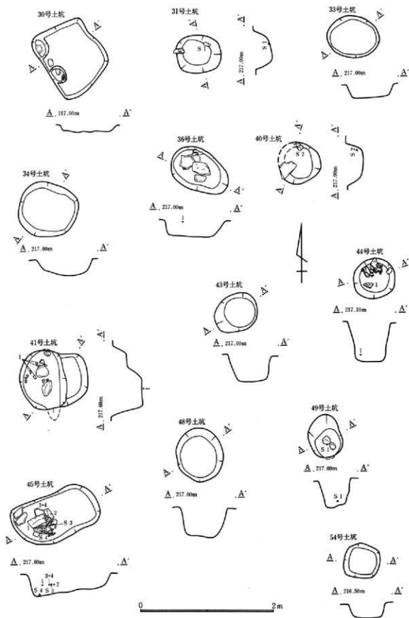
第347図 土坑遺構図
