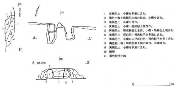
第293図 56号住居跡 カマド
