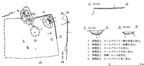
第308図 64号住居跡
