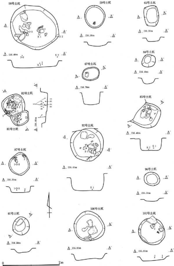
第348圖 土坑遺構圖
