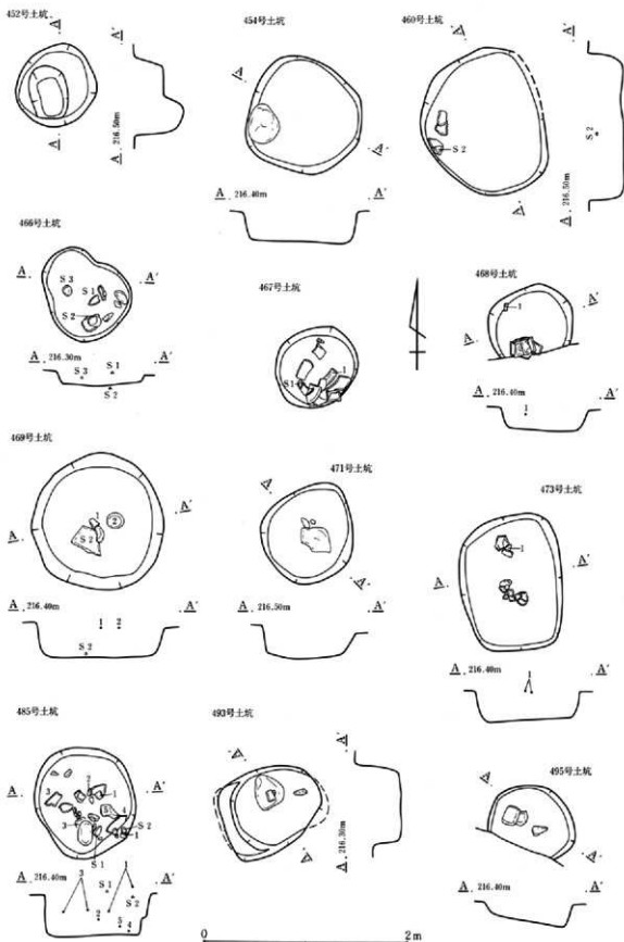
第361図 土坑遺構図
