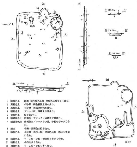
第288図 54号住居跡
