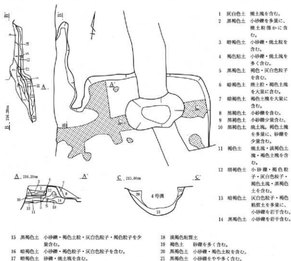
第326図 80号住居跡 カマド
