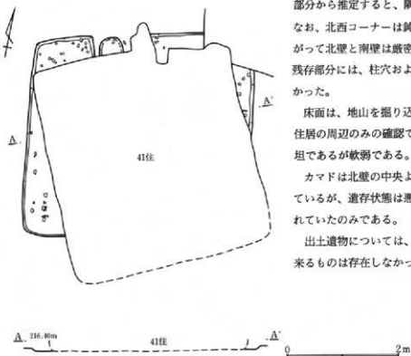
第324図 77号住居跡
