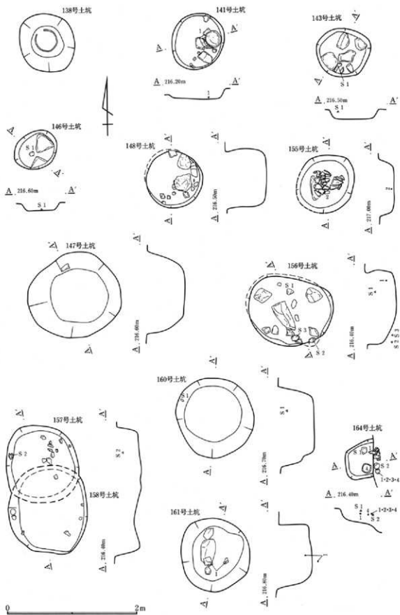
第350図 土坑遺構図
