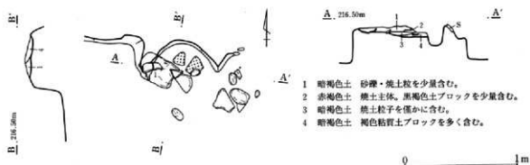
第286図 53号住居跡 カマド
