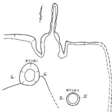
第296図 57号住居跡 カマド及び床下土坑
