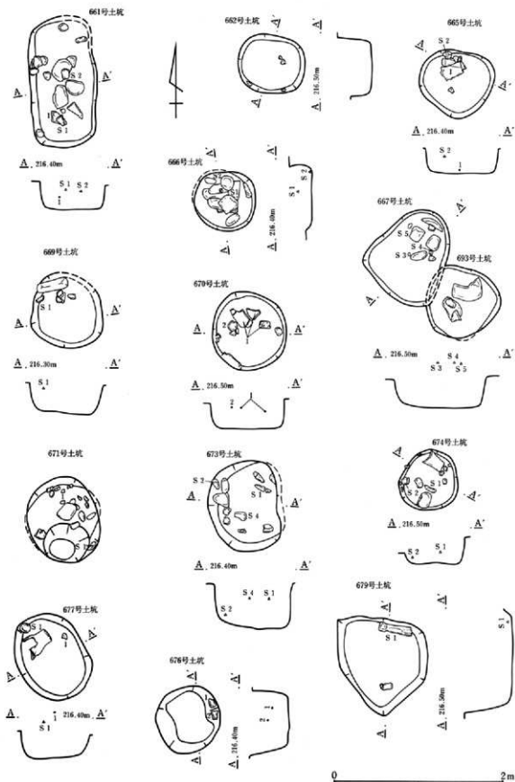
第369図 土坑遺構図
