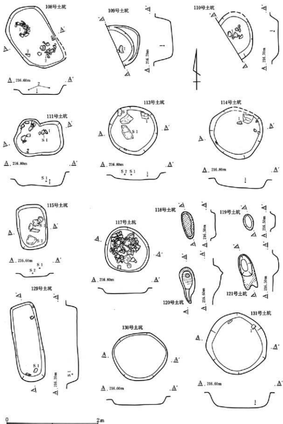
第349図 土坑遺構図
