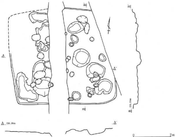
第333図 86号住居跡 掘り方
