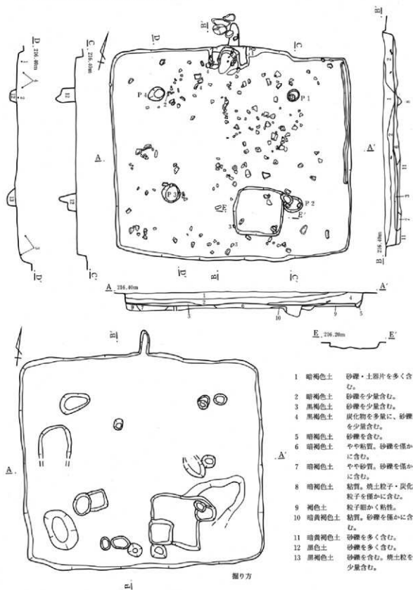
第305図 63号住居跡
