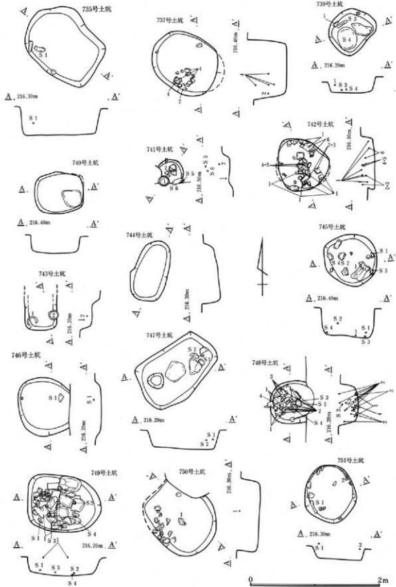
第372圖 土坑遺構圖
