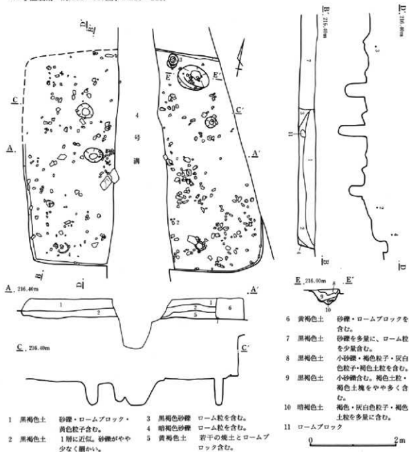
第332図 86号住居跡
