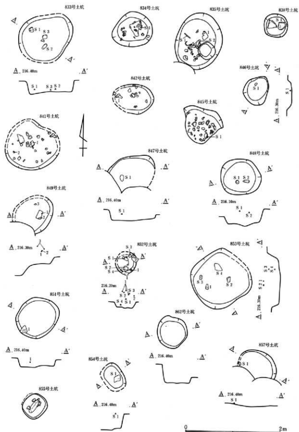
第375図 土坑遺構図
