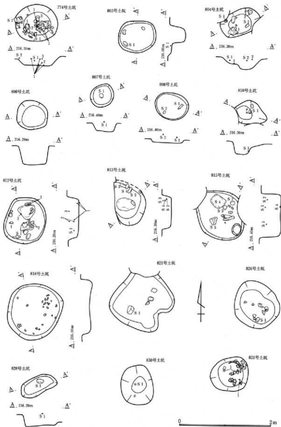
第374图 土坑遺構図
