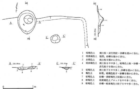
第341図 89号住居跡 カマド
