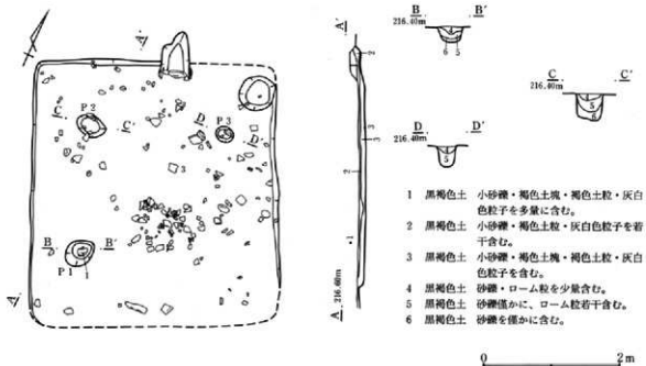
第264図 41号住居跡
