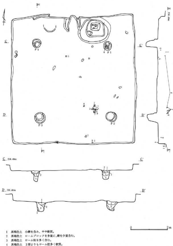
第276図 47号住居跡
