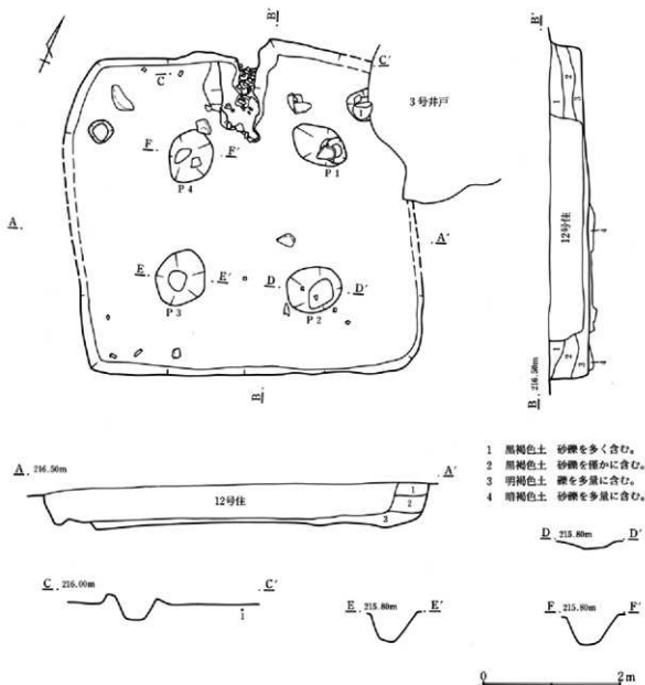
第282図 51号住居跡
