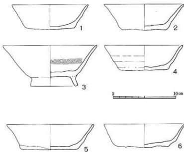
第38图 下綾垣遺跡1号墓主体部出土土器实测图
