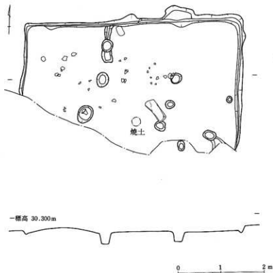
第7図 今村遺跡3号堅穴実測図 (1/50)
