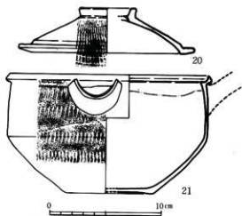
第10回 土器・陶磁器実測図（2）
