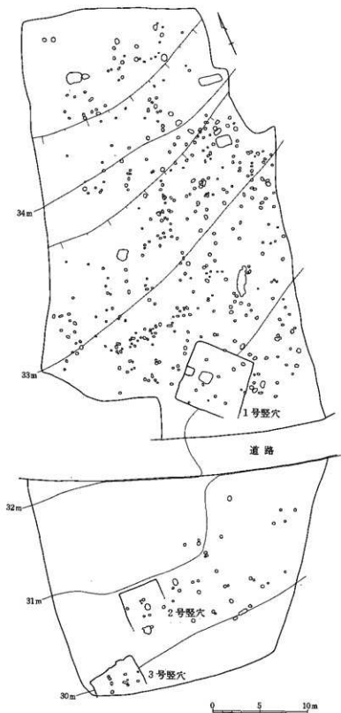
第2圖 今村遺跡遺構配置圖 (1/400)
