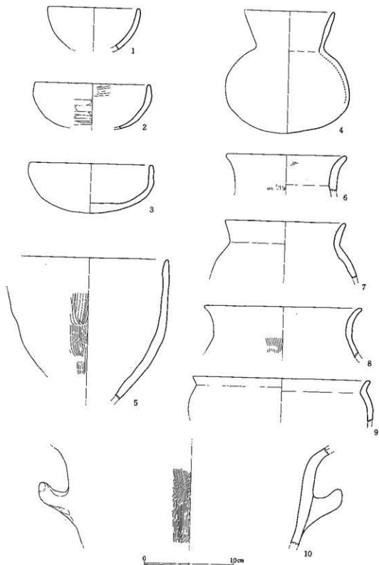
第4回 今村遺跡1号竪穴出土遺物実測図(寸)
