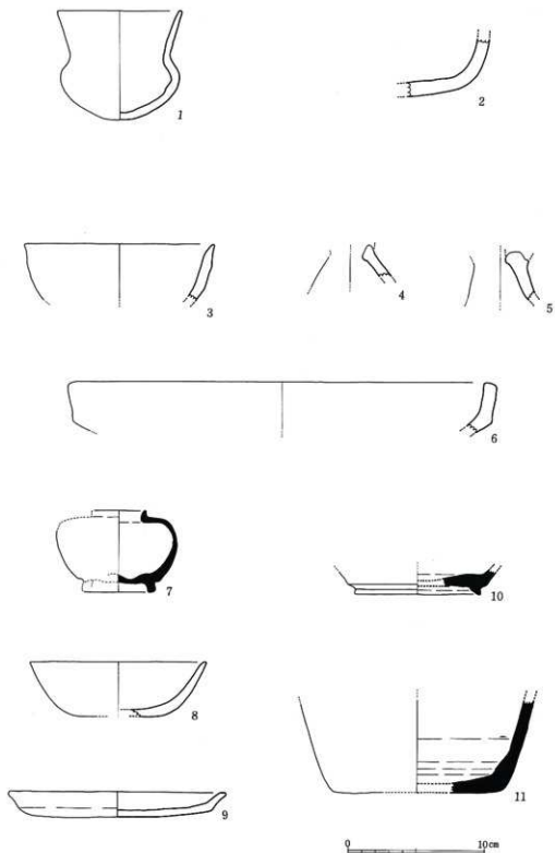
第8図 今村遺跡3号竪穴 (1.2) 今村一括出土遺物(3~11)実測図(1/5)
