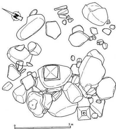
第3圖 角塔婆实测图
