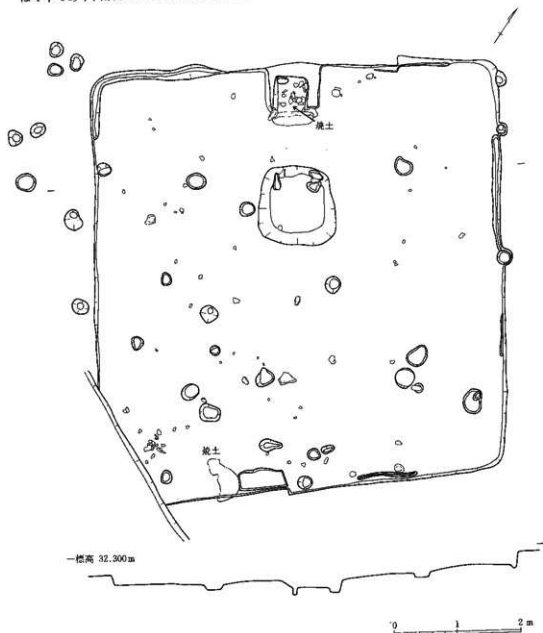
第3図 今村遺跡1号竪穴実測図 (1/60)
