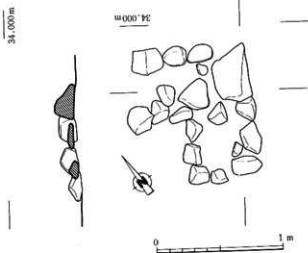
第7図 集石2実測図
