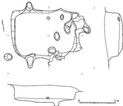
第58図 成田尾遺跡12号土坑実測図 (1/30)
