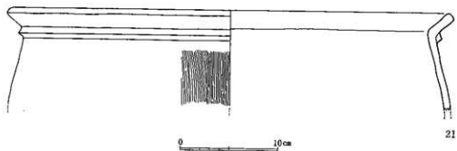
第31图 成田尾遺跡2号整穴出土遺物実測図(十)
