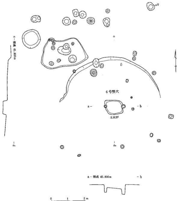
第35図 成田尾遺跡6号竪穴実測図 (1/400)
