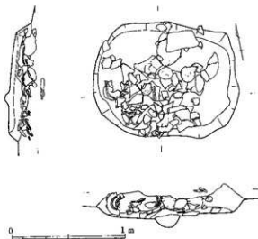
第79図 成田尾遺跡34号土坑実測図(1/30)
