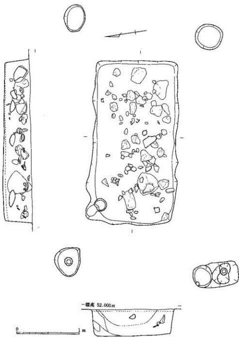
第49図 成田尾遺跡5号土坑実測図 (1/30)
