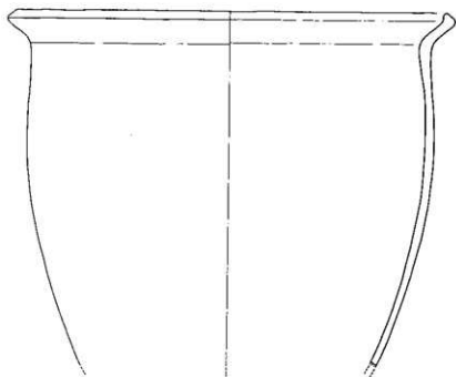
第44図 成田尾遺跡4号小児土器棺墓実測図(1/20)
