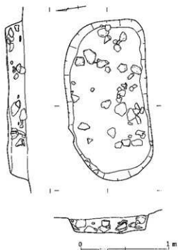
第52图 成田尾遺跡6号土坑実測図 (1/30)
