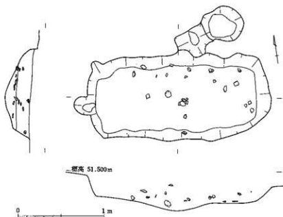
第55図 成田尾道跡9号土坑実測図 ( \frac{1}{30} )
