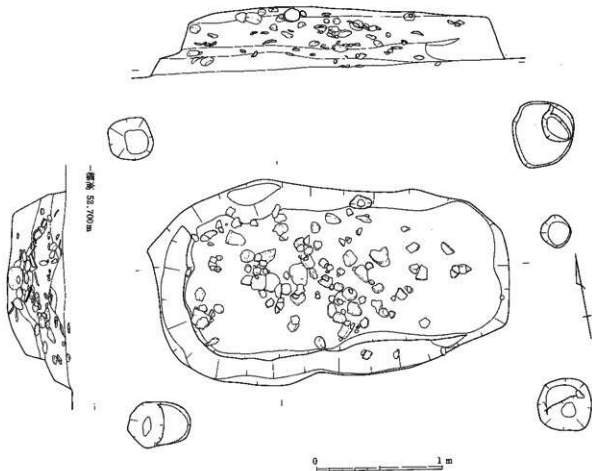
第46図 成田尾遺跡1号土坑実測図(1/30)
