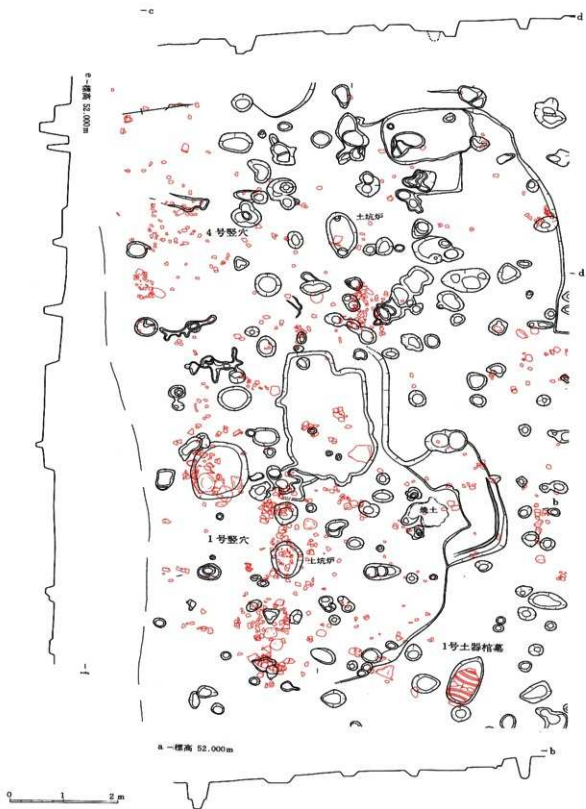
第4图 成田尾遺跡1号、4号整穴実測图 (1/500)
