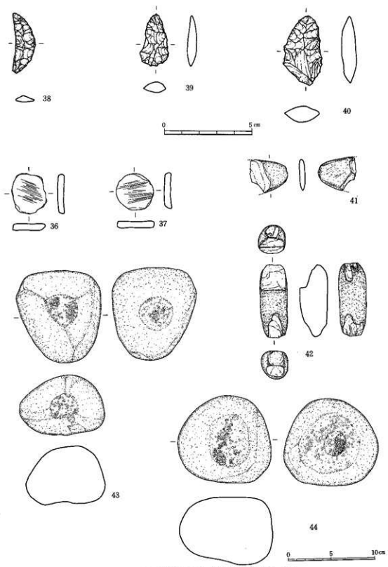
第15圖 成田尾遺跡1号竪穴出土遺物実測圖(子・十)
