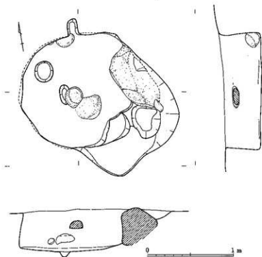
第76図 成田尾遺跡30号土坑実測図 (1/30)
