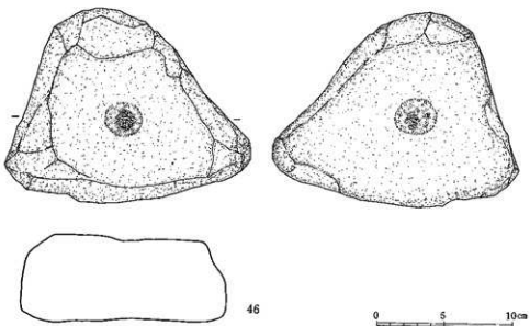
第26圖 成田尾遺跡4号壘穴出土遺物実測図 (1/4・1/2)
