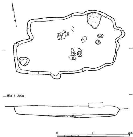
第68図 成田尾遺跡19号土坑実測図 (1/30)
