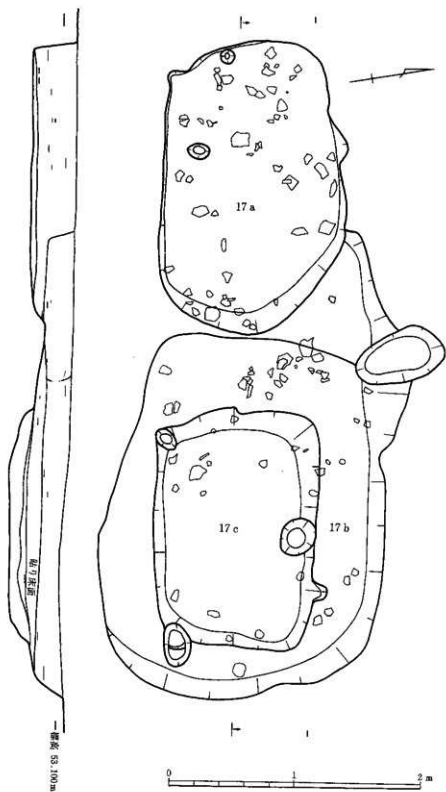
第65図 成田尾遺跡 17a、17b、17c号土坑実測図 (1/50)
