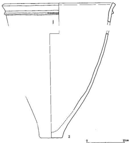
第43図 成田尾遺跡2号小児土器棺墓土器棺実測図(1/2)
