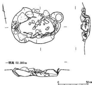
第41図 成田尾遺跡2号小児土器棺墓実測図 (1/20)
