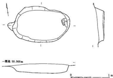
第62図 成田尾遺跡15号土坑実測図 ( \frac{1}{30} )
