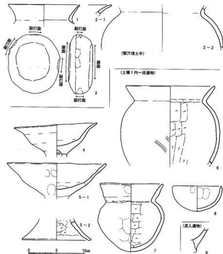
第5図 4号竪穴遺物出土遺物実測図 (1/3)
