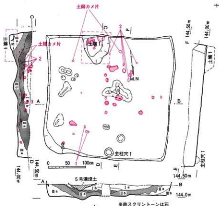
第3図 4号壑穴建物 平面図・断面土層図 (1/50)
