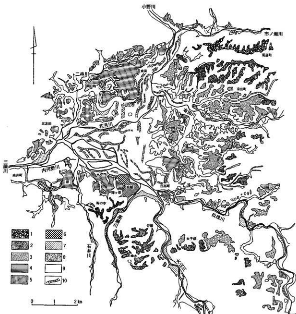
第3図 日田盆地の地形分類図 (千田昇「日田・玖珠地域の地形」第2図を再トレス)
