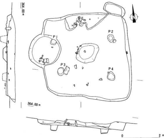
第16図 原田遺跡3号住居跡実測図
