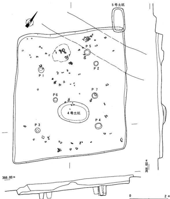
第38図 原田遺跡8号住居跡実測図
