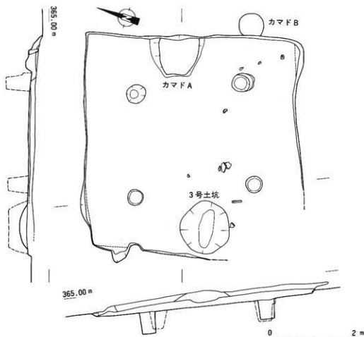
第31図 原田遺跡6号住居跡実測図
