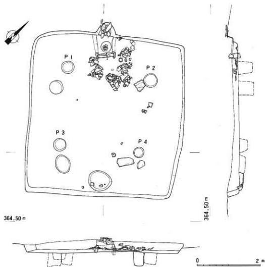
第19図 原田遺跡4号住居跡実測図
