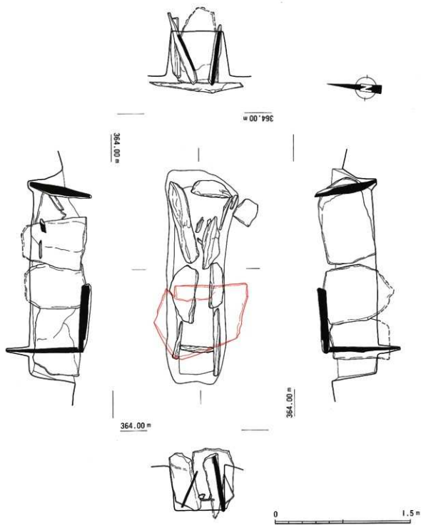
第76图 玖珠SA地区遗迹群1号石棺实测图
