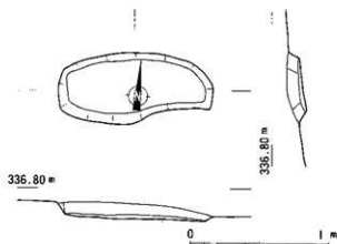
第90図 谷ノ瀬遺跡4号上坑実測図
