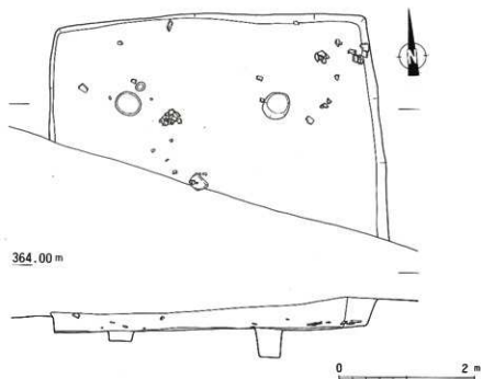
第14图 原田遺跡2号住居跡実測図
