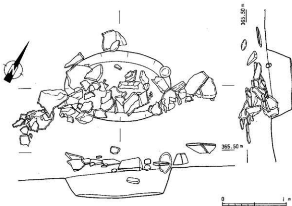
第58図 原田遺跡5号土坑実測図
