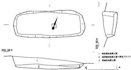
第94図 谷ノ瀬遺跡8号土坑実測図
