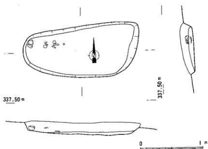
第89图 谷ノ瀬遺跡3号土坑実測図
