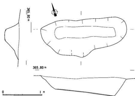
第60図 原田遺跡7号土坑実測図
