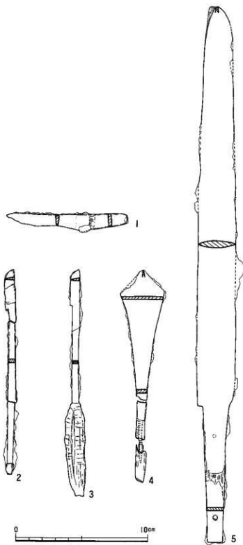
第72図 岩塚古墳出土土遺物実測図
