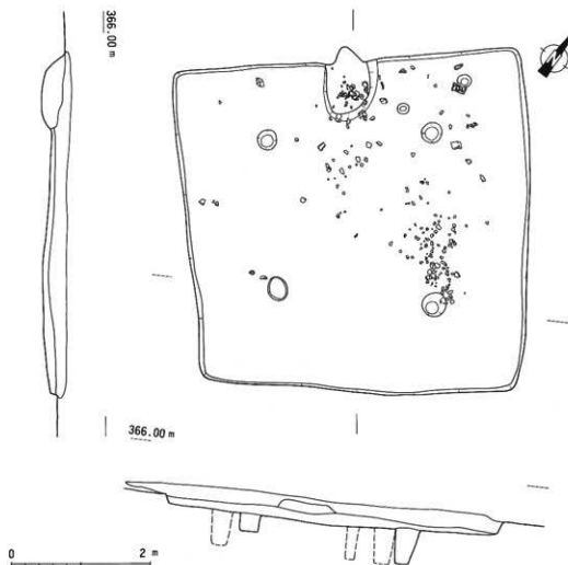
第35図 原田遺跡7号住居跡実測図
