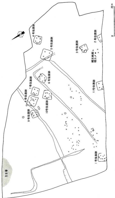
第10図 原田遺跡遺構配置図
