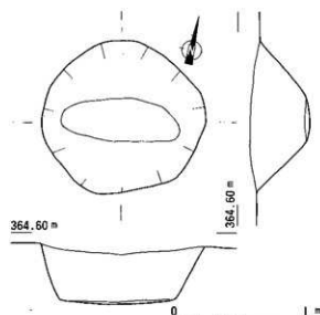
第56図 原田遺跡3号土坑実測図
