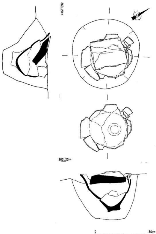
第51図 原田遺跡埋甕遺構実測図
