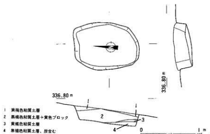
第92図 谷ノ瀬遺跡6号上坑実測図
