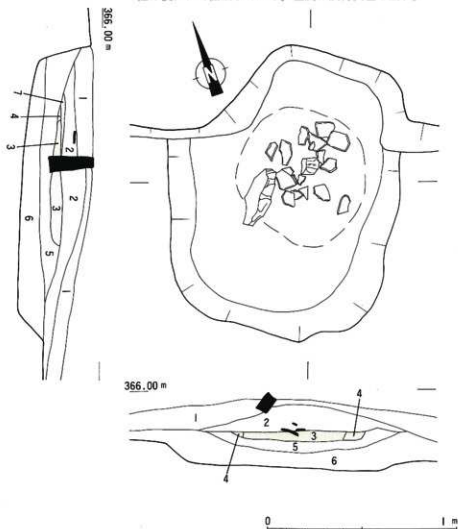
第43図 原田遺跡9号住居跡カマド実測図
