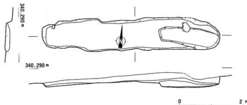
第86図 谷ノ瀬遺跡1号炭窯跡実測図
