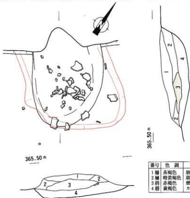
第36図 原田遺跡7号住居跡カマド実測図
