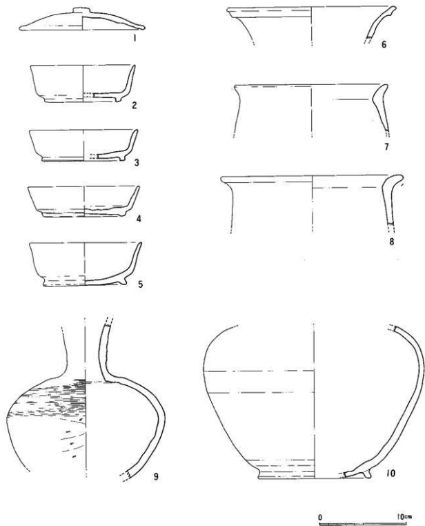
第7图 堂陶遗址1号竖穴出土器物实测图
