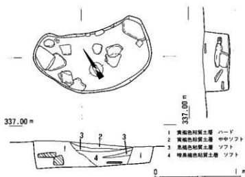
第93図 谷ノ瀬遺跡7号土坑実測図
