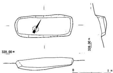
第91図 谷ノ瀬遺跡5号上坑実測図
