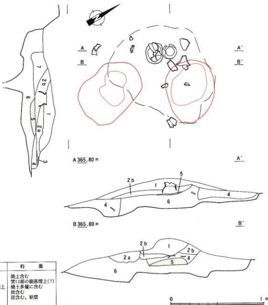
第39図 原田遺跡8号住居跡カマド実測図
