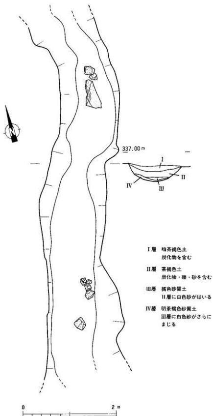
第96図 谷ノ瀬遺跡溝状遺構実測図
