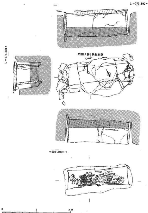
第71图 岩塚古墳主体部实测图
