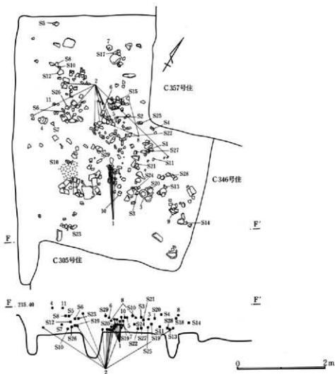
第315図 C361号住居跡(1)
