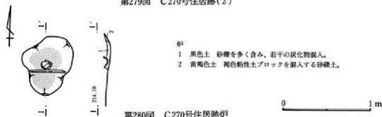
第280図 C270号住居跡炉
