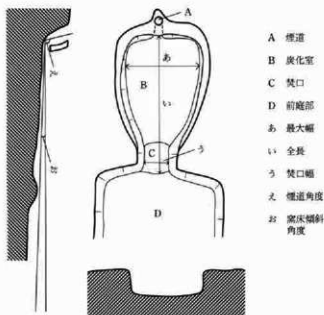
図10 炭焼窯計測ポイント図
