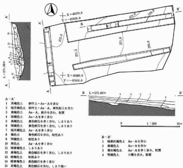
図24 調査区東半トレンチ平・断面図
