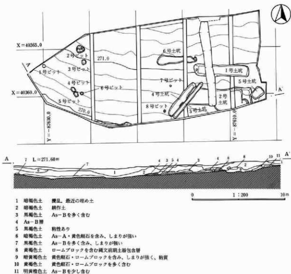
図25 調査区西半平・断面図
