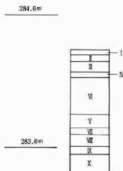
図43 基本層序図
