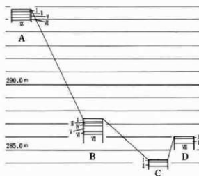
図32 基本層序図
