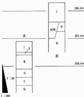
図7 基本層序図
