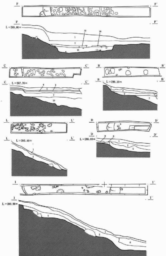
図35 トレンチ平・断面図(2)
