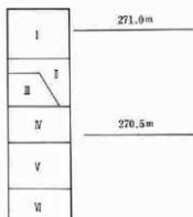
図22 基本層序図
