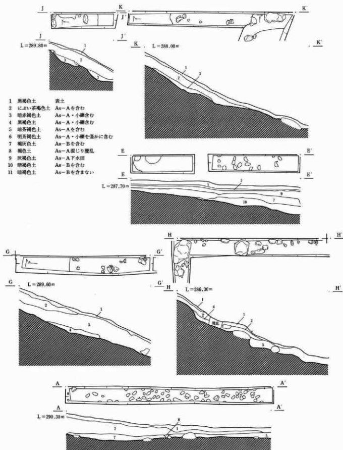
図34 トレンチ平・断面図(1)
