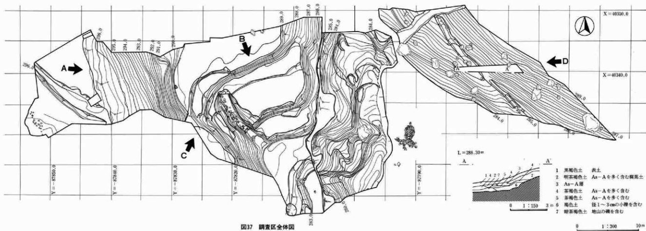
図37 調査区全体図
