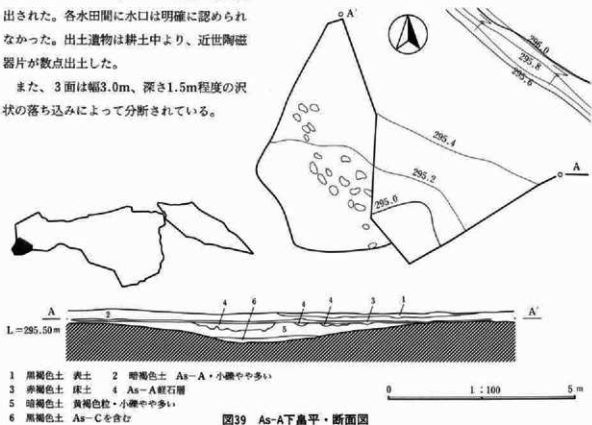
図39 As-A下畠平・断面図
