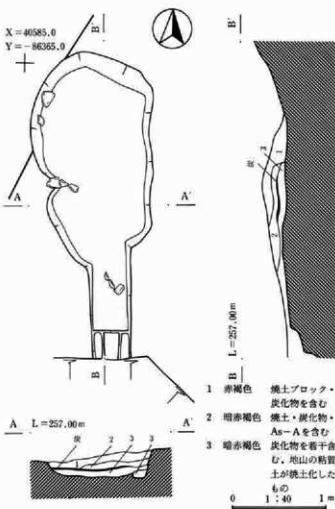
図11 炭焼窯平・断面図
