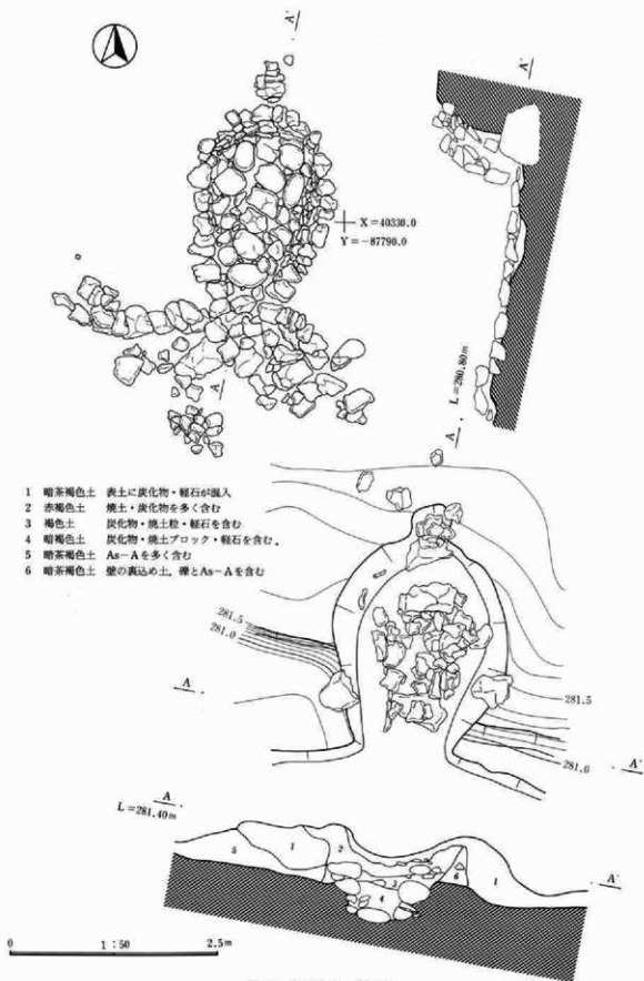
図38 炭焼窯平・断面図
