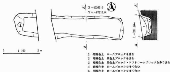
図26 1号土坑平・断面図
