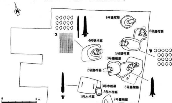
吹上遺跡 6次調査遺構配置図
