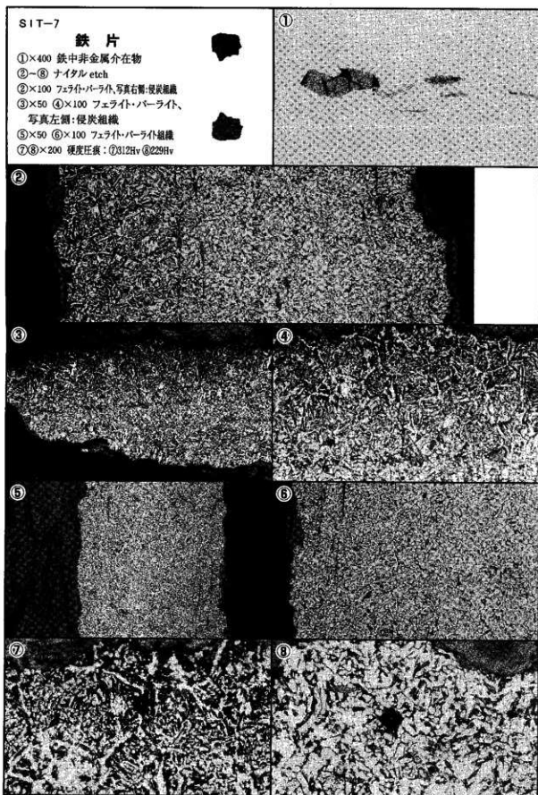
Photo.6 鉄片の顕微鏡組織
