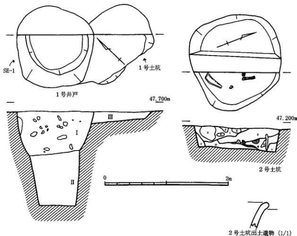
第20図 Ⅰ区1・2号土坑、1号井戸実測図 (1/30) 及び出土遺物実測図 (1/1)
