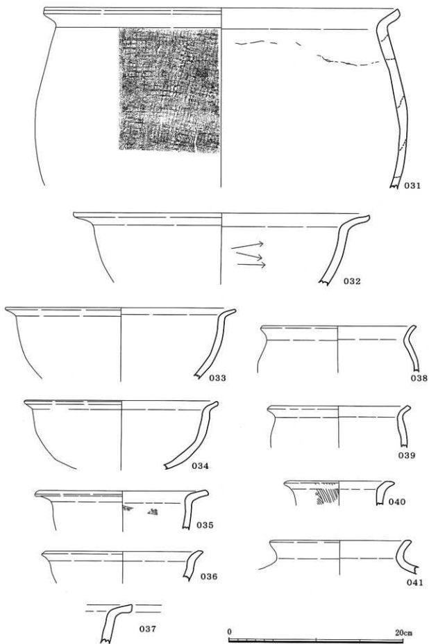
第35图 二目川遺跡Ⅱ区SH2出土遺物実測図(3)
