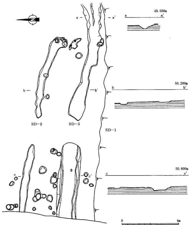
第45図 二目川遺跡Ⅱ区溝状遺構実測図
