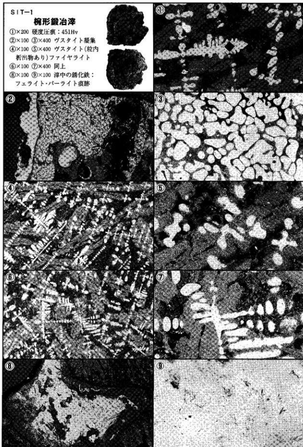
Photo.1 梘形鍛冶滓の顕微鏡組織
