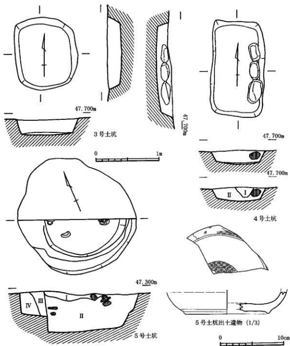
第21図 I区3～5号土坑実測図(1/30)及び土遺物実測図(1/3)
