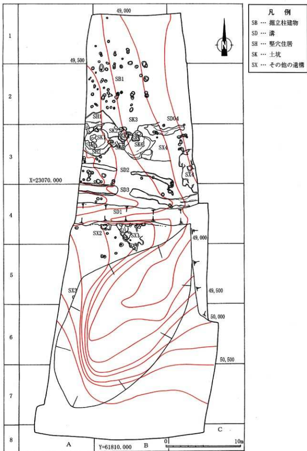
第26図 二目川遺跡Ⅱ区遺構配置図
