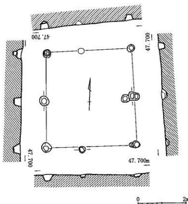
第19図 1号掘立柱建物実測図(1/80)
