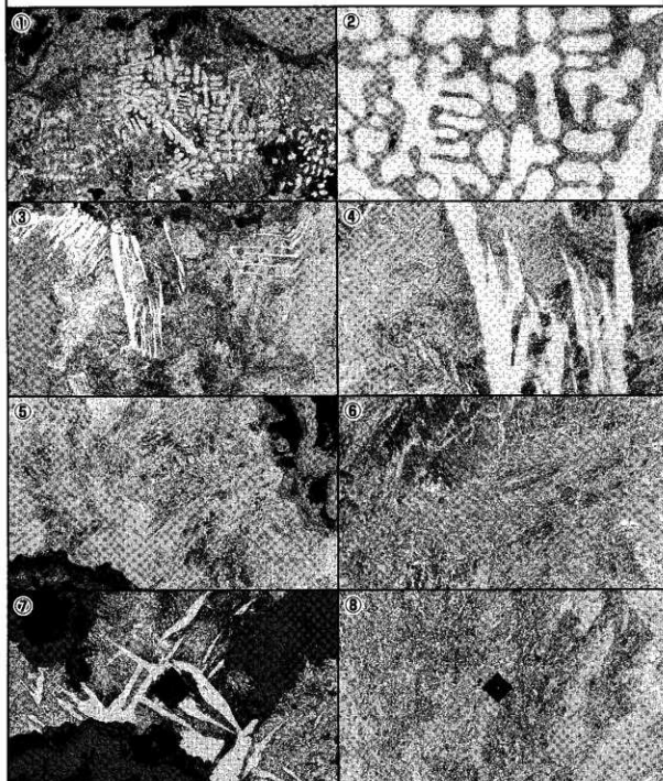
Photo.5 含鉄梔形鐵冶滓の顕微鏡組織
