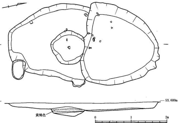
第10図 2号不定形土坑実測図 (1/30)
