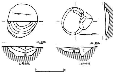
第24図 I区12・13号土坑実測図(1/30)
