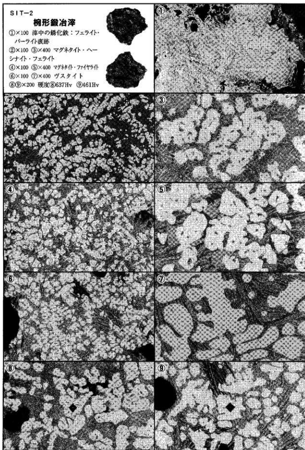
Photo.2 梶形鍛冶滓の顕微鏡組織
