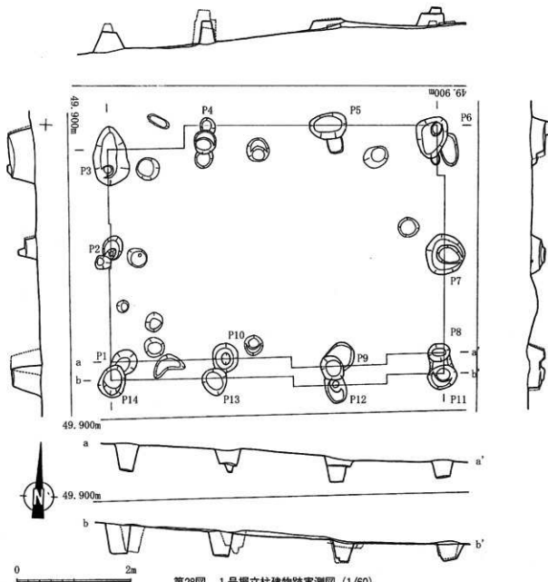
第28図 1号掘立柱建物跡実測図 (1/60)
