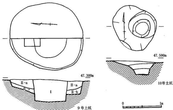
第23図 I区9～10号土坑実測図 (1/30)
