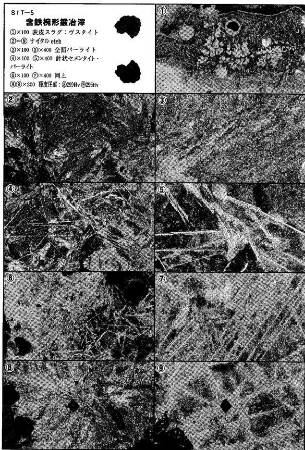
Photo.4 含鉄梔形鐵冶滓の顯微鏡組織
