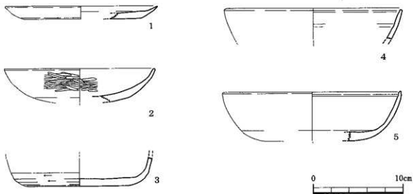
第11図 2号不定形土坑出土遺物実測図 (1/30)
