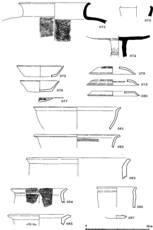
第41图 二目川遺跡Ⅱ区SK6出土遺物実測図
