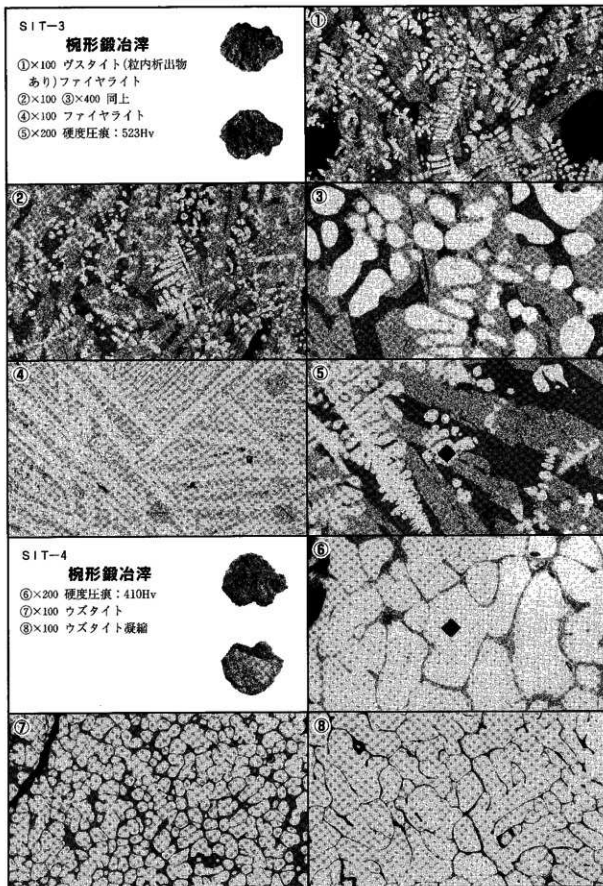
Photo.3 梘形鐵冶滓の顕微鏡組織
