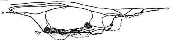
第30図 二目川遺跡Ⅱ区北側土坑群土層断面及び実測図(1)
