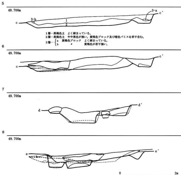
第31図 二目川遺跡Ⅱ区北側土坑群土層断面及び実測図(2)
