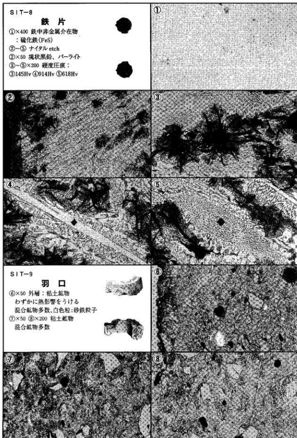
Photo.7 鉄片・羽口の顕微鏡組織
