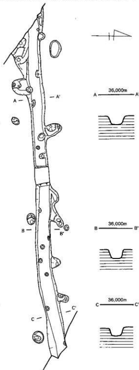
第15図 1号溝状遺構 (1/40)
