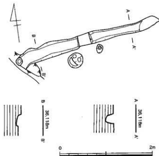
第16図 2号溝状遺構 (1/40)
