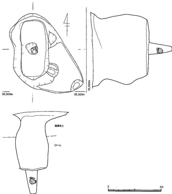
第20図 3号陥し穴実測図
