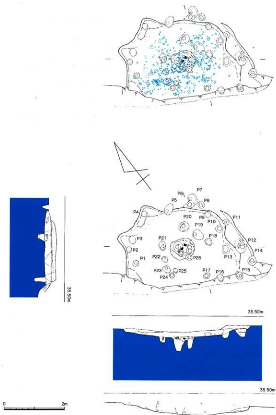
第4图 1号整穴住居跡実測図
