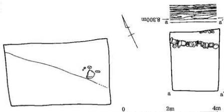
第68図 8区 平面図と南壁土層図
