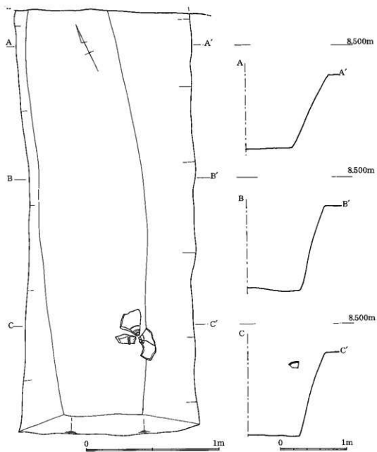
第25図 3区 SD1平断面図
