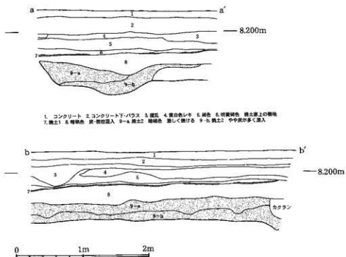
第127図 16区 南壁・西壁土層図
