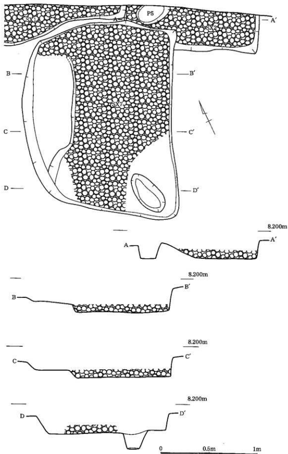
第14图 1区 SX7·SX2平断面图
