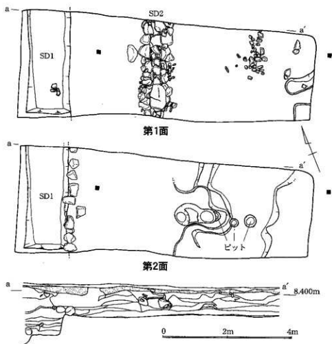
第24図 3区 平面図（第1・2面）と北壁土層図
