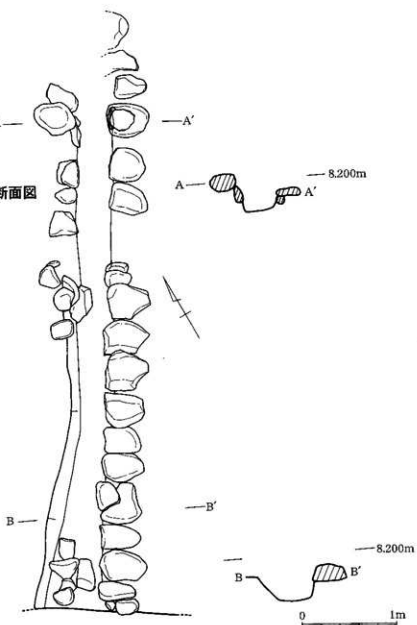
第116-3图 15区 南北石列第3面 平断面图
