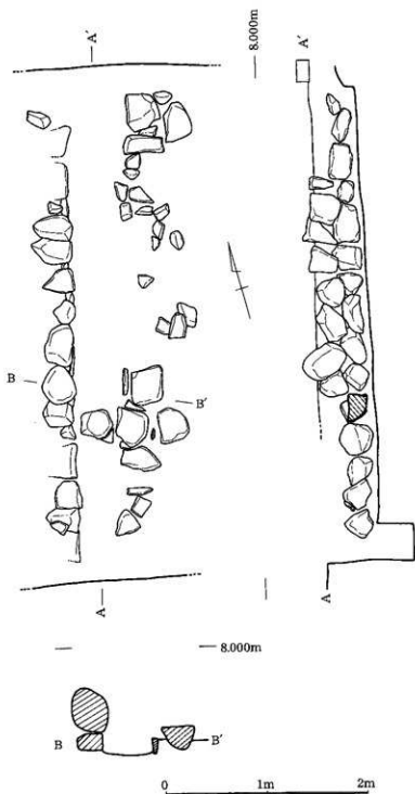
第75図 9区SD1平面図
