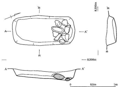
第60図 7区 SK2平断面図
