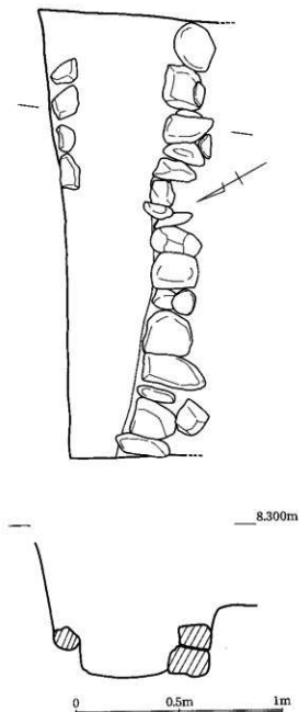
第69図 8区 SD1断面図
