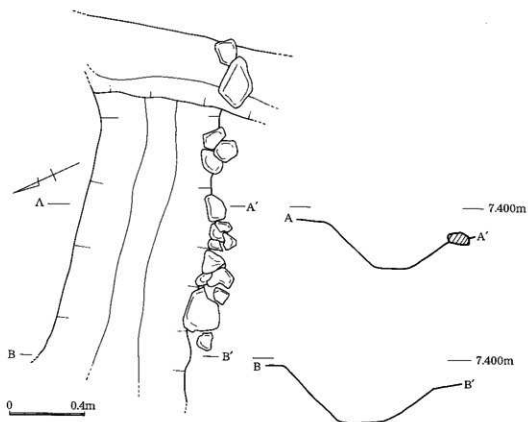
第111図 14区 石列平面図
