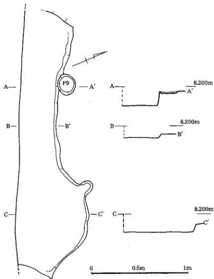
第6図 1区 SD2平面図
