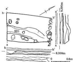
第125図 16区 平面図と南・西壁の土層図
