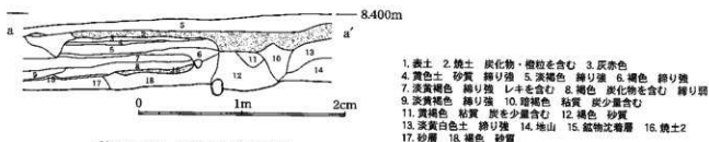
第66-1図 7区 西壁土層図
