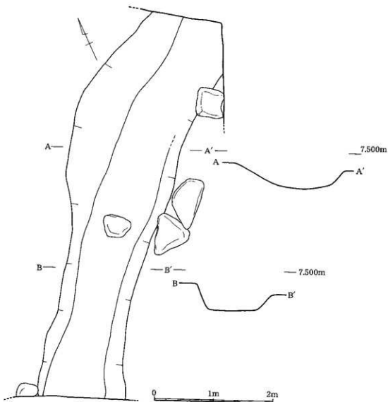
第126図 16区 SD1平断面図
