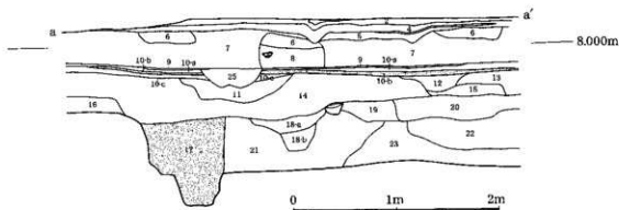
第107図 14区 東壁土層図
