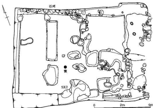
第93図 12区 平面図
