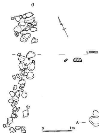
第116-2图 15区 南北石列第2面 平断面图
