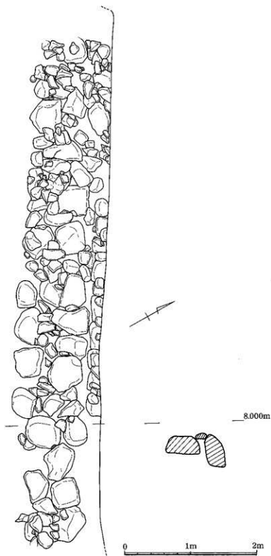
第118-2图 15区 東西石列第2面平面図
