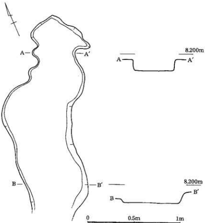
第4図 1区 SD1 断面図
