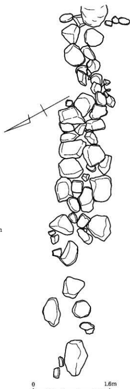
第118-3图 15区 東西石列第3面平面図
