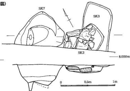
第86図 10区 SK 2・3・7断面図
