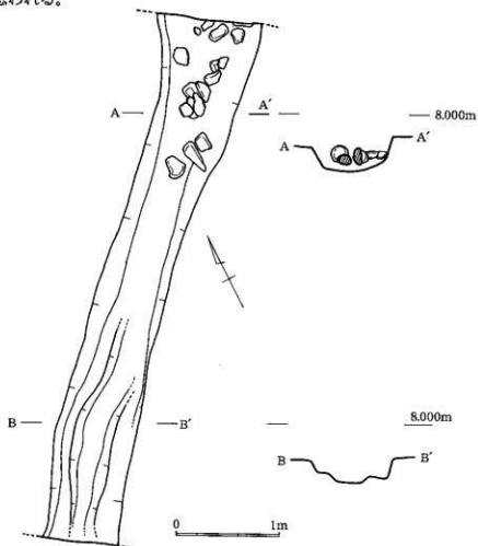
第84図 10区 SD1平断面図
