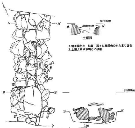
第27図 SD2 断面図
