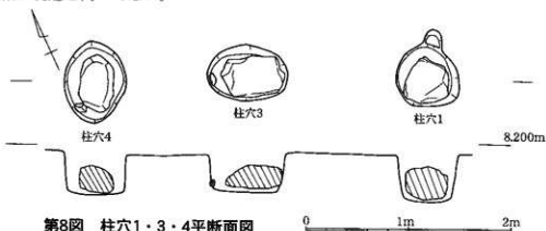
第8図 柱穴1・3・4平断面図
