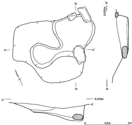
第43図 5区 焼土坑平面図
