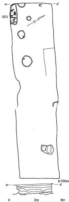
第19図 2区 平面図・東壁土層図
