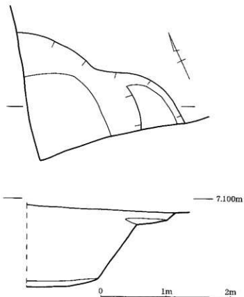
第77図 9区 2面 SK2 (焼土坑) 平断面図
