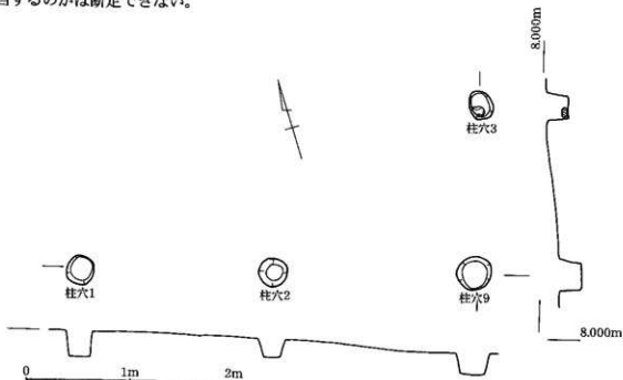
第53図 6区 柱穴1・2・9・3 平面図
