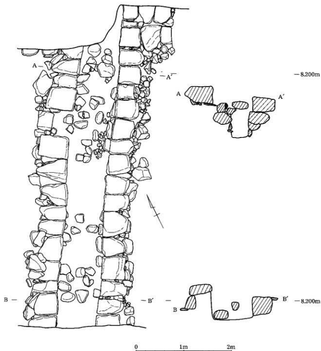
第116-1図 15区 南北石列第1面 平断面図
