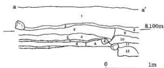
第37図 4区 西壁土層図
