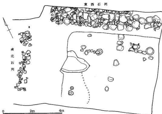
第121図 15区 第2面平面図
