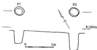
第36図 4区 柱穴平面断面図
