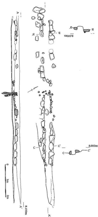
第45図 5区 SD2平面図
