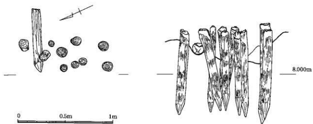
第46図 5区 SD1の下で検出した杭 平断面図
