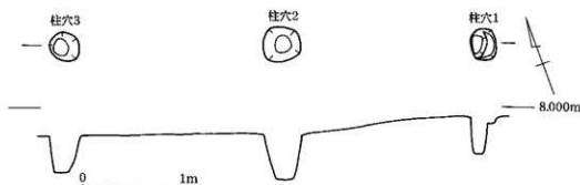
第64図 7区 柱穴平面図
