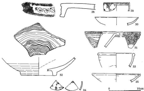
第114-3図 14区 その他の遺物
