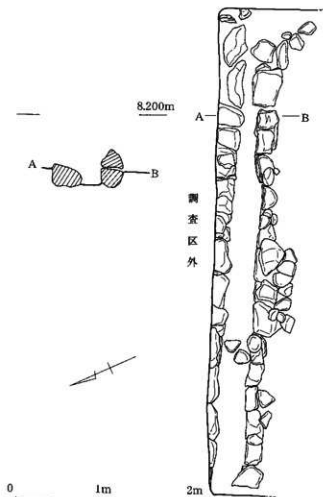
第33図 4区 SD1平断面図
