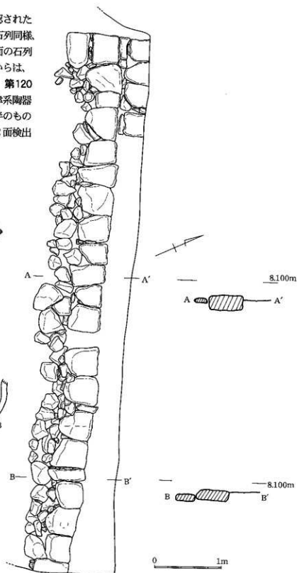
第118-1図 15区 東西石列第1面断面図
