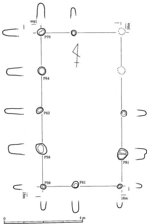
第4図 SB 1の平面図
