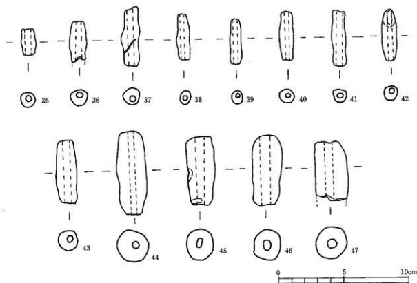
第12図 出土遺物実測図 (1/2)
