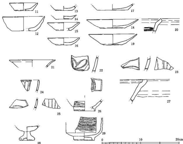
第10図 出土遺物実測図 (1/3)
