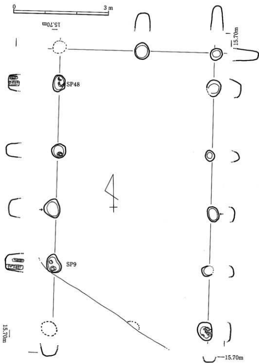
第5図 SB2の平面図
