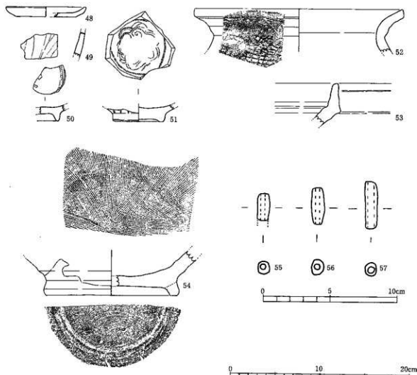
第13図 出土遺物実測図 (1/3)(土鍾は1/2)
