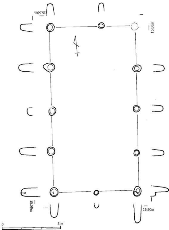
第6図 SB3の平面図
