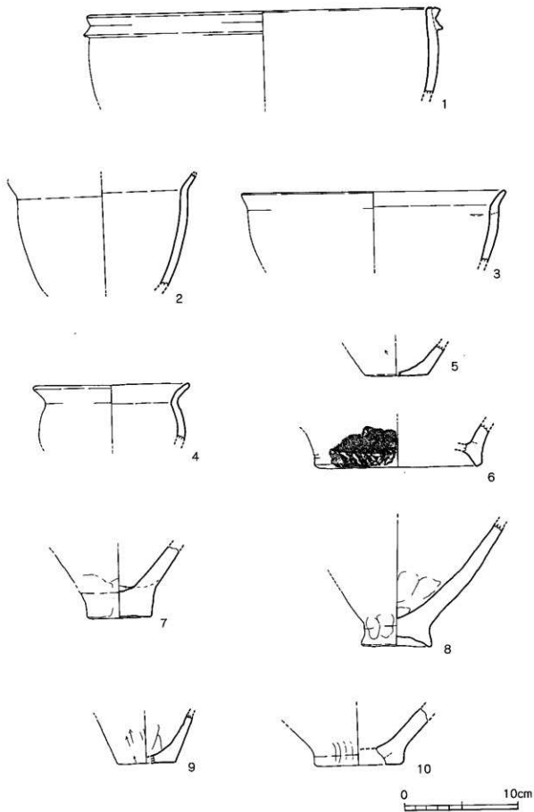
第18图 東大濠遺跡A地区 出土遺物 実測図(2)
