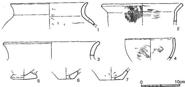
第9図 東大道遺跡A地区 SDO2出土遺物実測図
