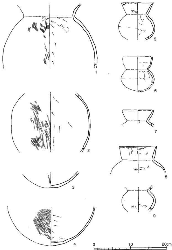
第12图 襄大道遗址A地区 住居跡(SX01)出土遺物 実測図2
