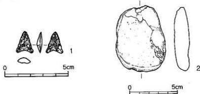
第8図 東大道遺跡A地区 SDO2出土石器実測図
