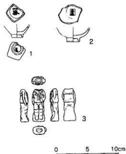
第22図 東大道遺跡A地区 出土遺物 実測図(6)
