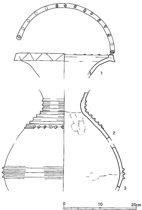
第19图 東大道遺跡A地区 出土弥生土器 実測図(3)
