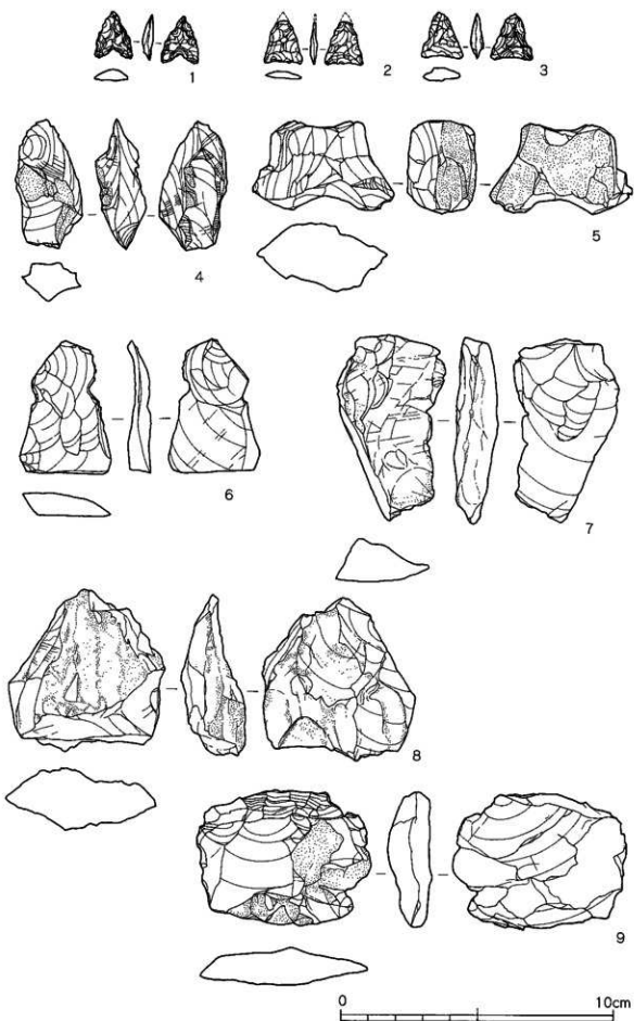
第15图 東大森遺跡A地区 出土石器 実測図(1)
