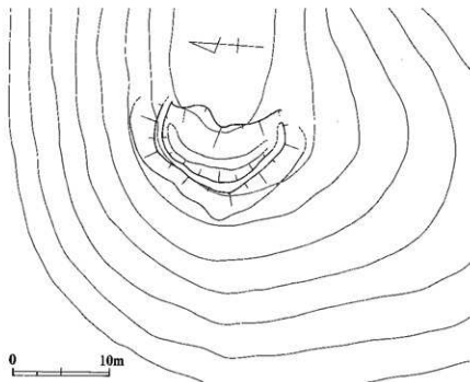
第10図 旗返峠台場1略測図 (S=1:400)
