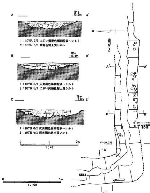
図95 3区SD14・15実測図
