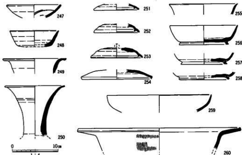
図88 長原2、4層出土遺物実測図
