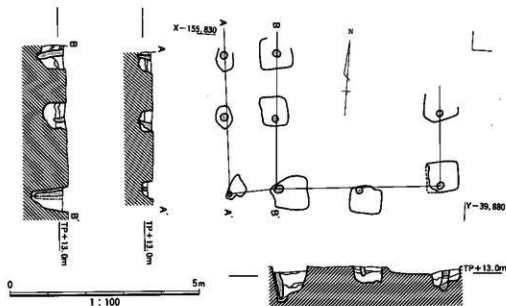
図91 1区SB01実測図
