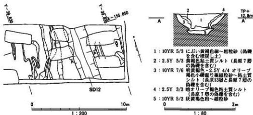
図94 2区SD12実測図
