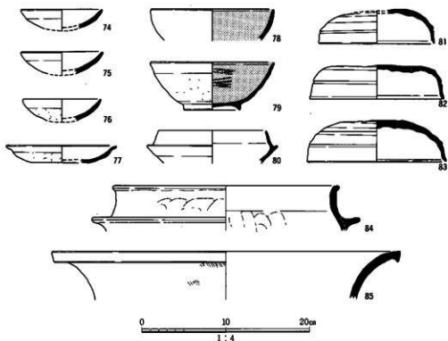
図45 長原4Biii、7層出土遺物実測図
