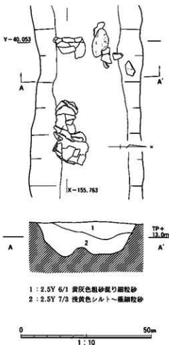
図105 SD18遺物出土状況図
