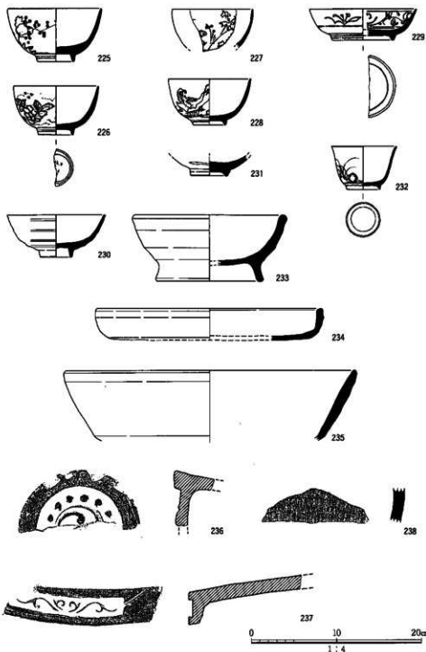
图84 SK05出土文物实测图
