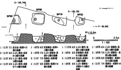
図102 柱列A実測図
