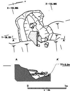
図18 SX902遺物出土状況図
