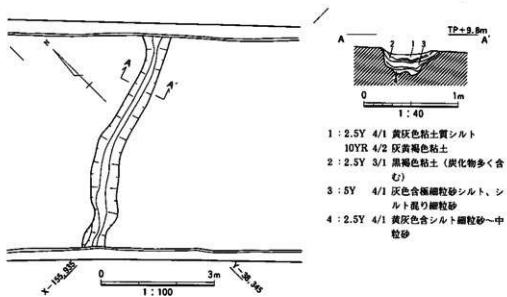
図37 1区SD601実測図
