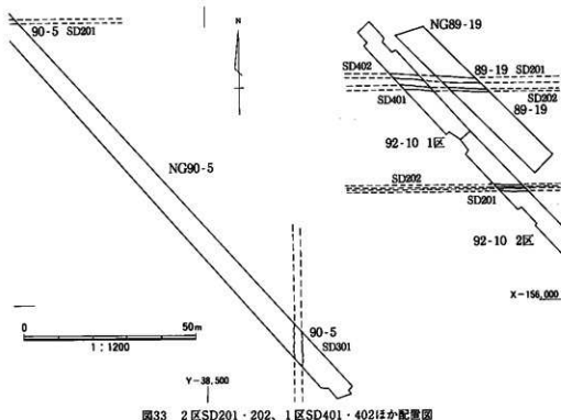
図33 2区SD201・202、1区SD401・402ほか配置図
