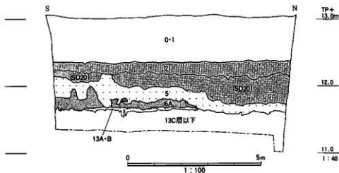
図77 南区西壁断面模式図
