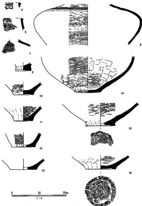
圖15 NR901出土遺物實測圖
