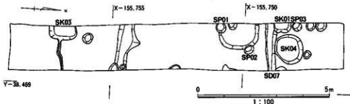
図59 長原4層下面検出遺構配置図
