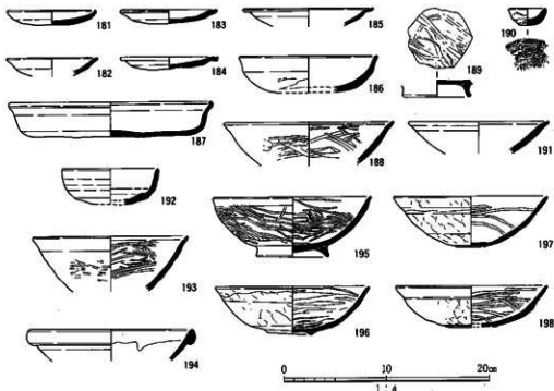
図69 SK02～04、SE01出土遺物実測図
