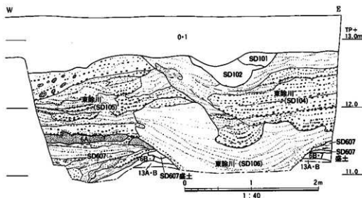
図76 北区北壁断面実測図
