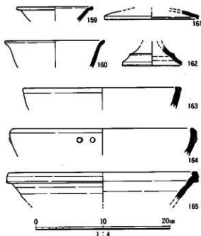
図62 長原2、4Bi層出土遺物実測図
