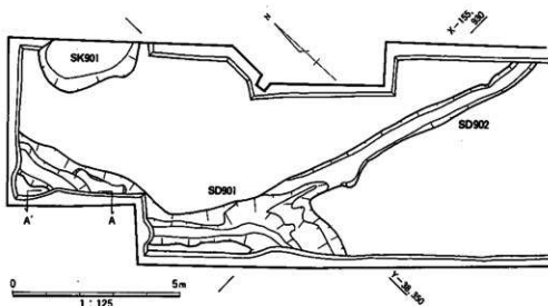
図38 1区SD901・902、SK901実測図
