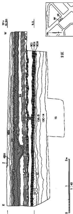
图61 南壁断面实测图
