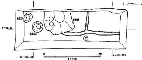
図70 2区SE02～04実測図
