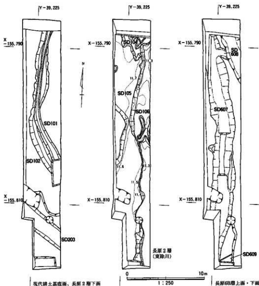
図78 北区遺構配置図
