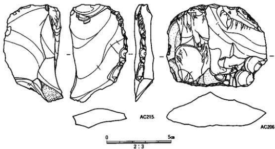
圖16 NR901出土石器遺物實測圖
