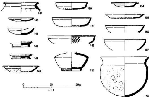
図60 SD07、SK01・03・04、SP01～03出土遺物実測図
