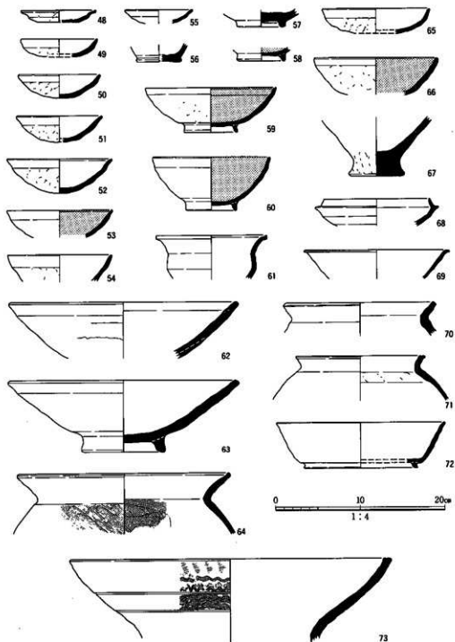
図44 長原4Bii、4Biii層出土遺物実測図
