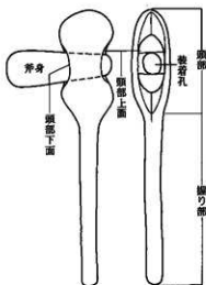
図108 縦斧直柄の各部名称
