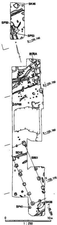
図100 長原4層基礎面検出遺構配置図
