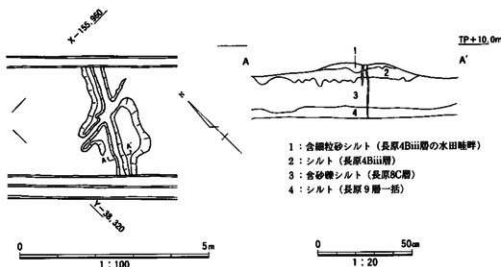
図36 2区SR401実測図
