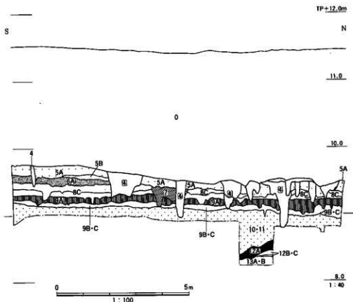
図57 西壁断面模式図
