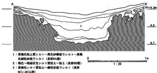
図39 1区SD901南壁断面実測図
