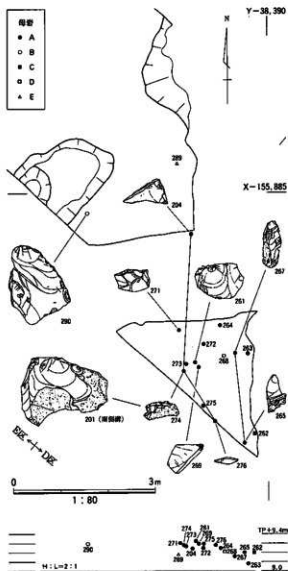
図22 LC1301出土石器遺物分布図
