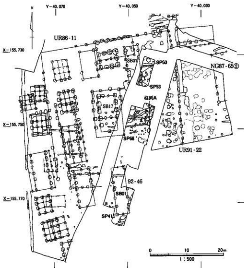
図107 掘立柱建物群検出状況図
