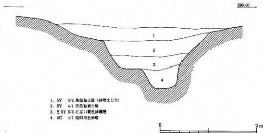
第10図 神宮寺西遺跡 溝1断面図
