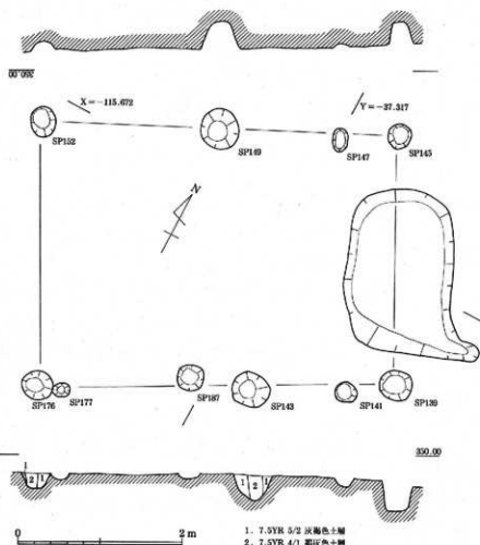
第22図 田能城跡 建物1平面・断面図
