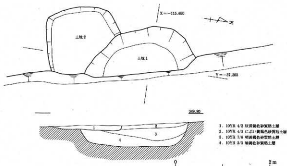
第17図 田能城跡 土坑1・2平面・断面図
