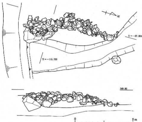
第15図 田能城跡 石垣平面・側面図
