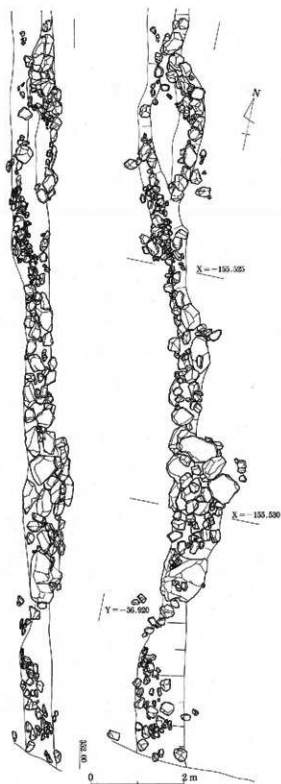
第30図 田能北遺跡 石垣1平面・断面図
