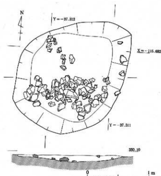
第23図 田能城跡 土坑4平面・断面図
