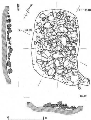
第24図 田能城跡 土坑5平面・断面図
