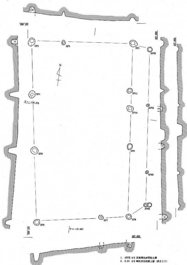
第5図 神宮寺西遺跡 建物1平面・断面図
