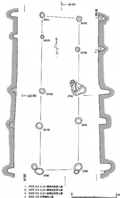
第29図 田能北遺跡 建物1平面・断面図
