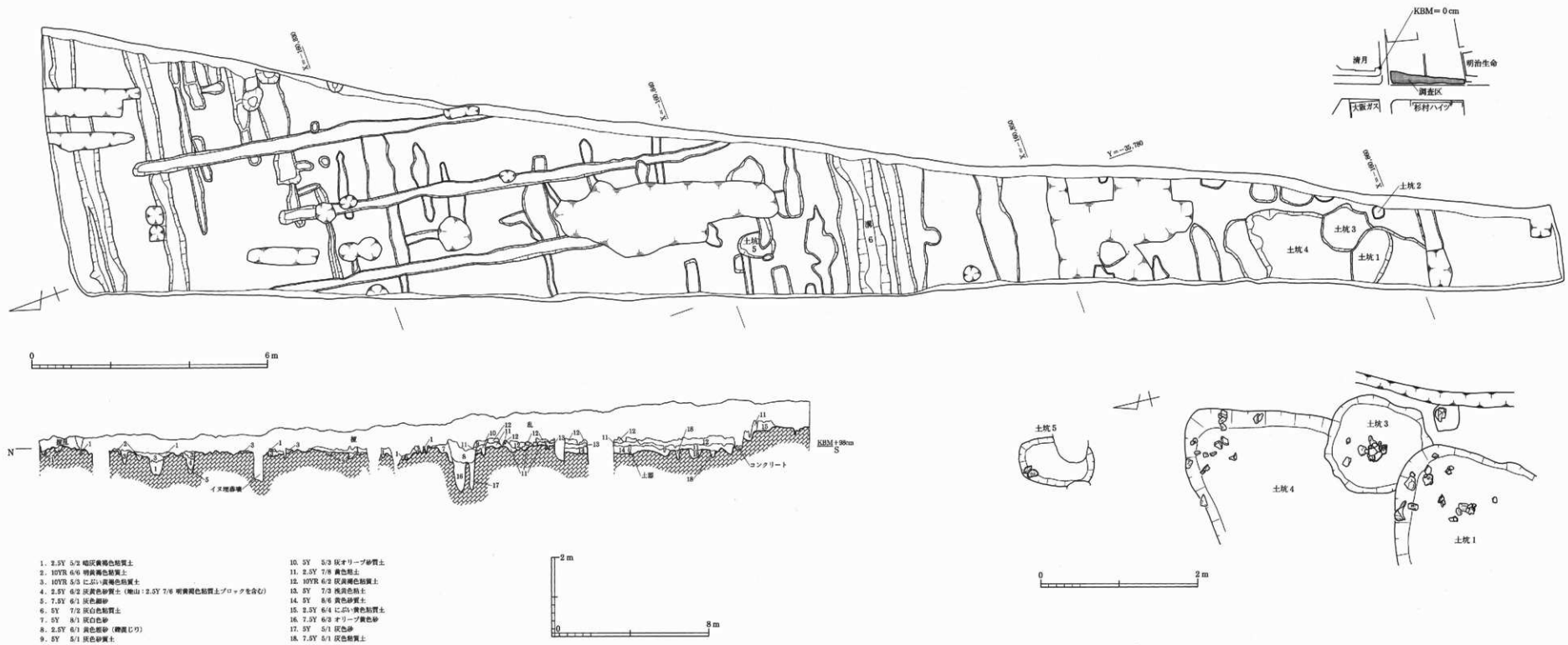
第3図 98年度調査区遺構平面図、西壁断面図、遺物出土状況
