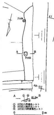
第29図 Pit 05・06 平・断面図
