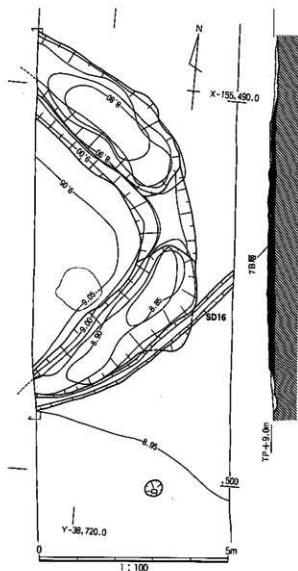
図157 148号墳平・断面図
