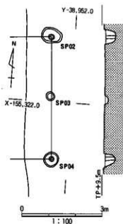
図85 SB01平・断面図
