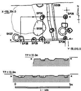
図89 SB05平・断面図
