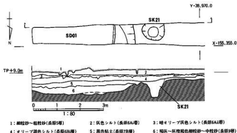
図54 IV区東調査区SD01・SK21平・断面図
