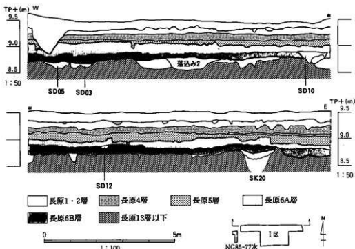
図49 中央地区Ⅰ区の層序
