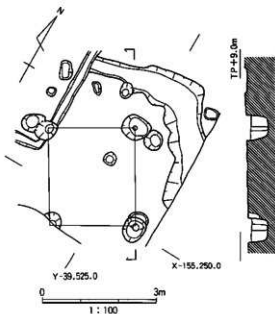
図27 SB05平・断面図
