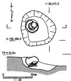
図98 SK27平・断面図
