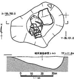
図132 SK01平・断面図
