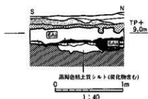
図66 SK10とその上層断面図
