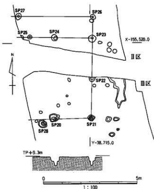
図196 SB04平・断面図
