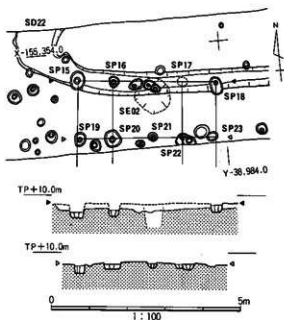
図88 SB04平・断面図
