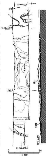
図159 149号墳平・断面図
