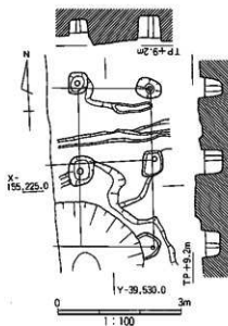
図31 SB09平・断面図
