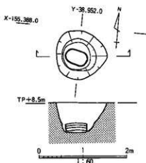
図95 SE03平・断面図
