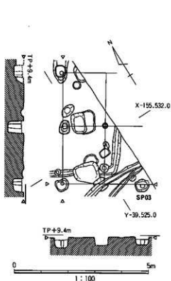
図29 SB07平・断面図
