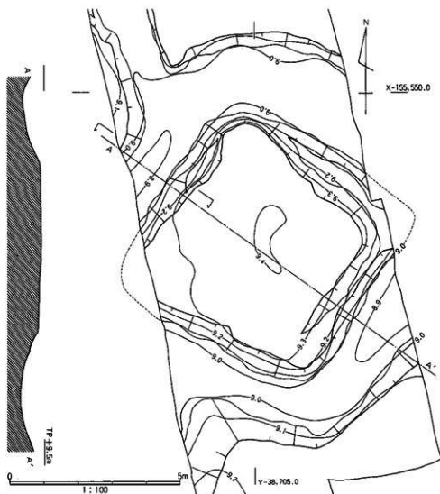
図171 151号墳平・断面図
