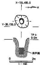
図200 SE01平・断面図
