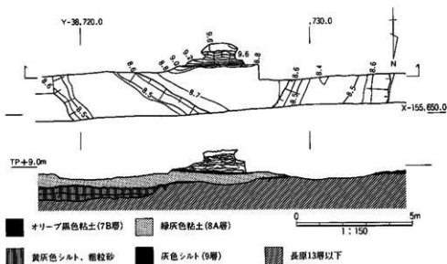
図173 152号墳平・断面図
