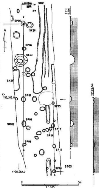
図86 SB02・03平・断面図
