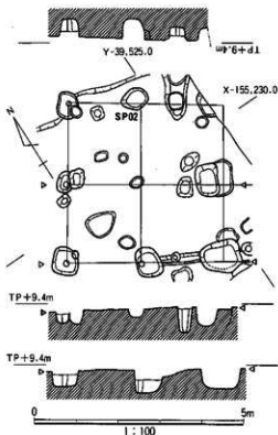
図30 SB08平・断面図
