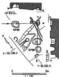
図28 SB06平・断面図
