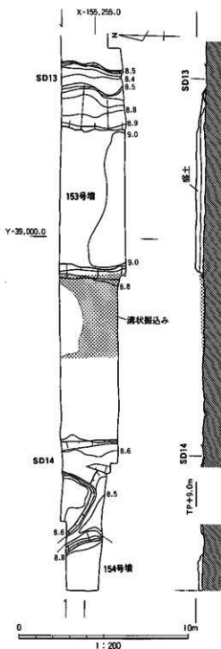
図61 153・154号墳平・断面図
