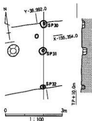
図90 SA01平・断面図
