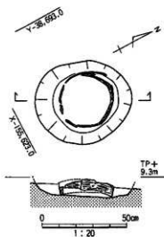
図208 SE08平・断面図
