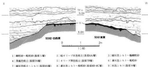
図144 SD01・02・03肩部断面図 (Ⅳ区南壁)
