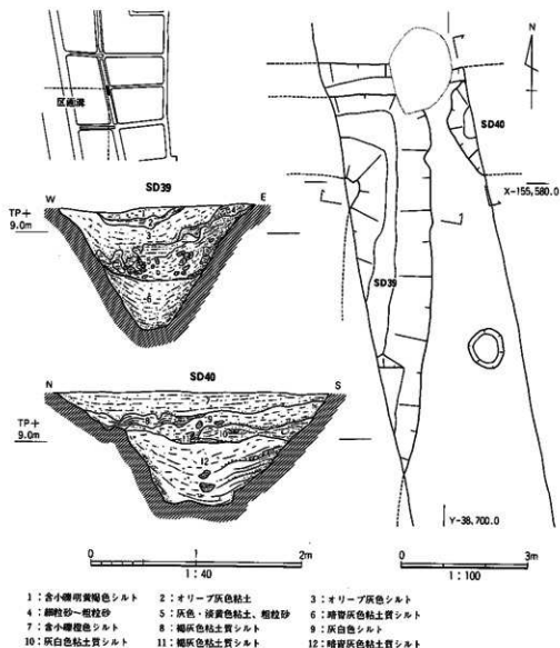
図210 SD39・40平・断面図
