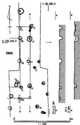
図129 SB03平・断面図 (08～19の数字は柱穴番号)
