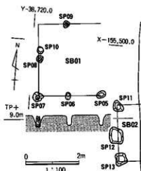
図194 SB01・02平・断面図
