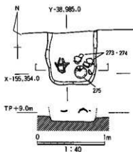
図70 SK23平・断面図
