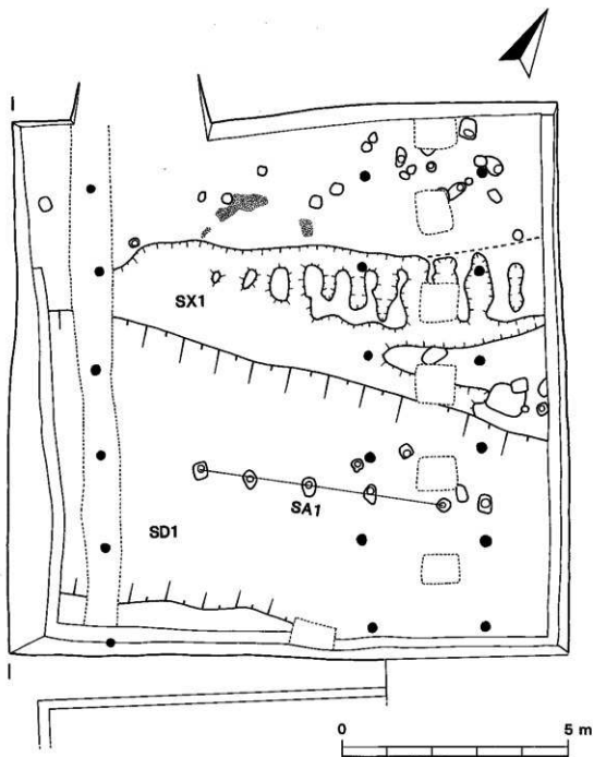
図4 第10次調査遺構全図
