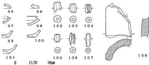
図11 SX1出土遺物（須恵器・土錘・瓦）
