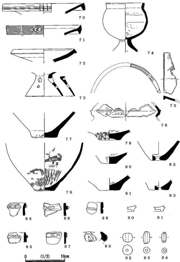
図10 SD1出土遺物（器台・その他）
