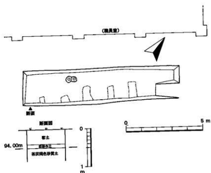
図17 T5 トレンチ遺構図
