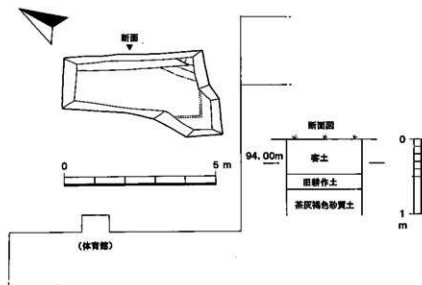
図14 T2トレンチ遺構図
