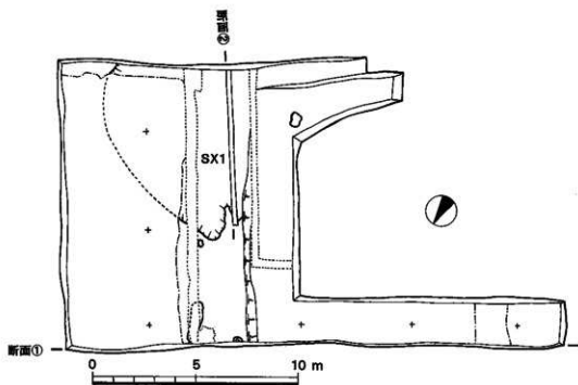
図18 T6トレンチ遺構図
