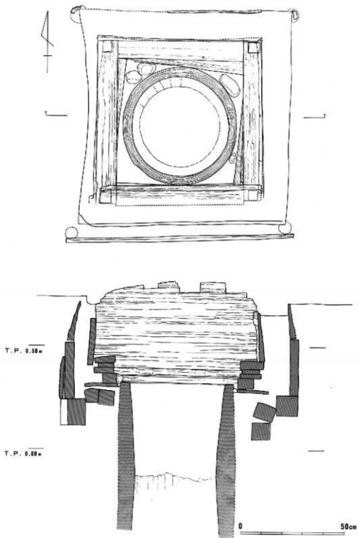
第26図 井戸2 平面図・断面図
