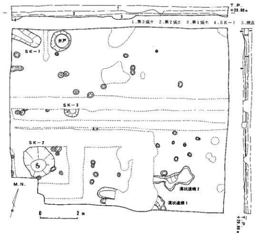
第44図 遺構平面図
