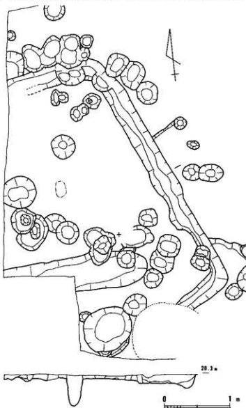
第9図 SH-5 平面図・断面図
