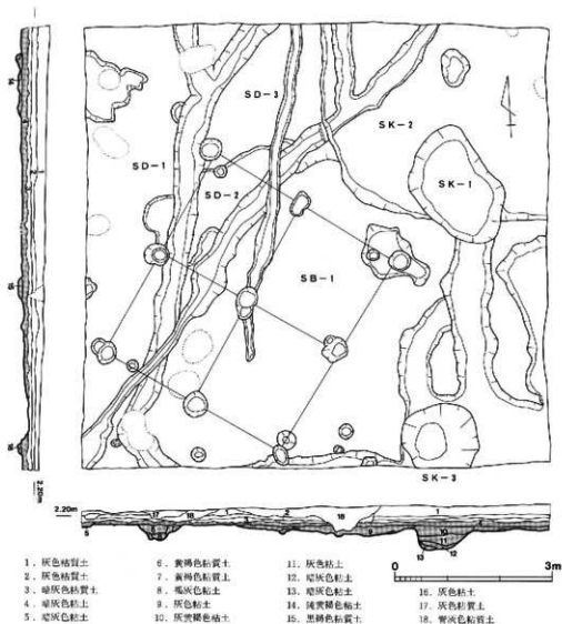
第4図 遺構平面図 (1:80)
