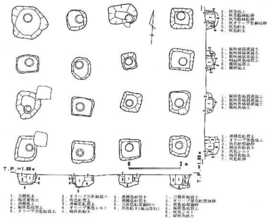
第22図 掘立柱建物1平面図・断面図
