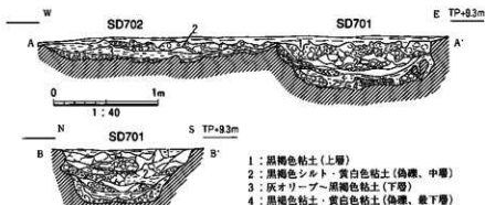
図88 SD701・702断面図
