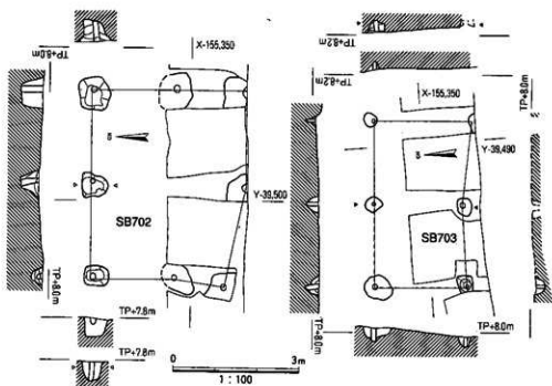
図23 SB702・703実測図
