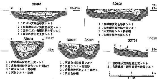
図46 古墳～奈良時代の遺構断面図
