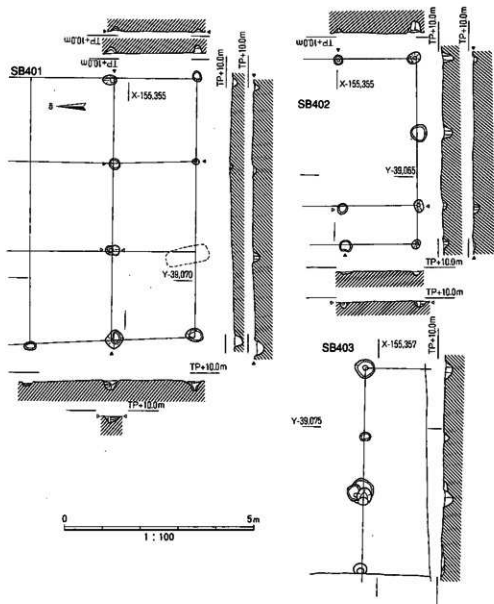
図84 平安時代の掘立柱建物実測図
