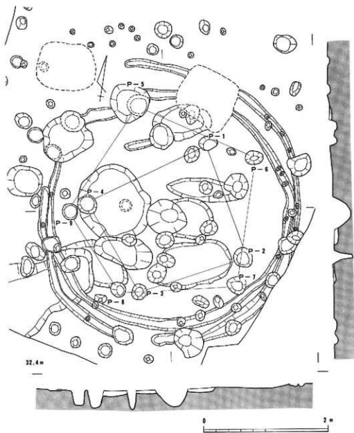
第5図 SB-1・2平面図
