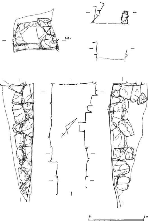
第18图 石室实测图
