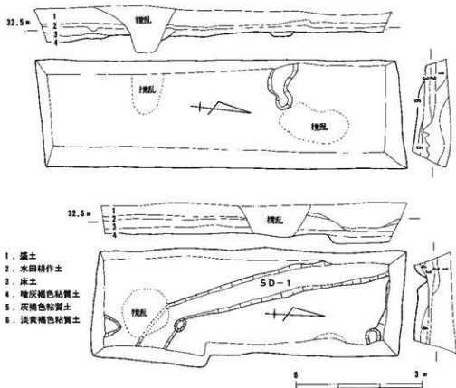
第15図 第1・2トレンチ平・断面図
