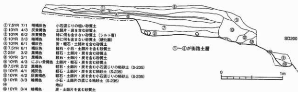
第50図 I-40東西方向断面図(土坑と万寿寺の堀と街路を示す) 1/30
