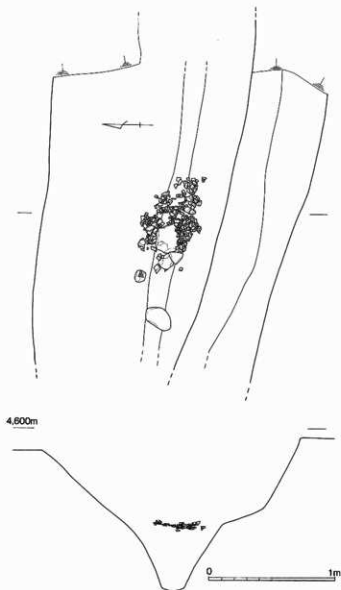
第108図 SD462及び出土遺物実測図 (1/30)
