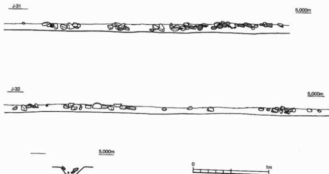
第95図 SD304側面図及び断面図(1/50)
