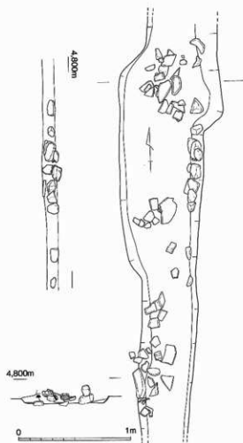
第94図 SD304の一部実測図(1/30)
