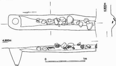
第106図 SD370・SP383実測図 (1/30)
