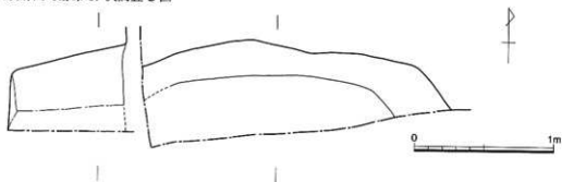
第361図 SK183実測図 (1/30)
