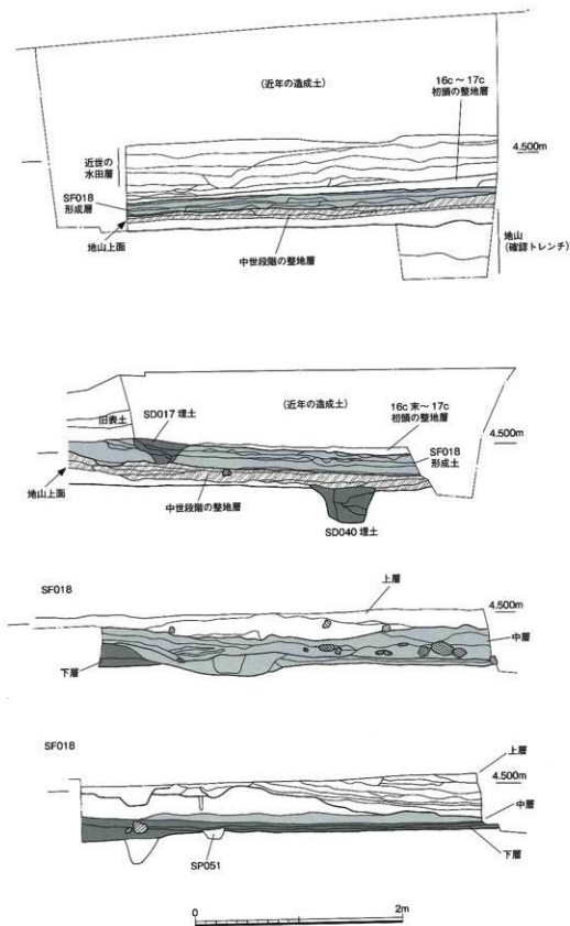
第 425 図 調査区土層実測図② (1/40)
