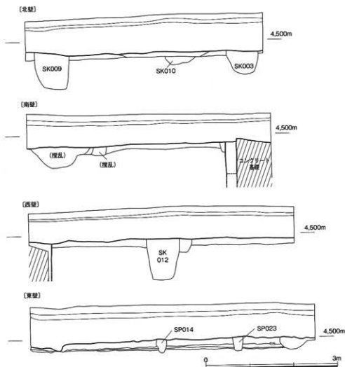
第413図 調査区土層実測図 (1/60)
