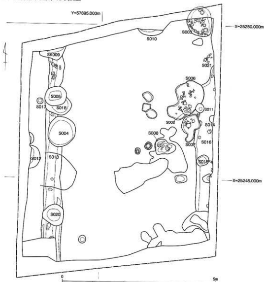
第412図 第78次調査区遺構配置図(1/60)
