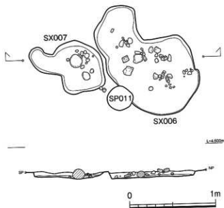
第418図 SX006・SX007実測図(1/30)
