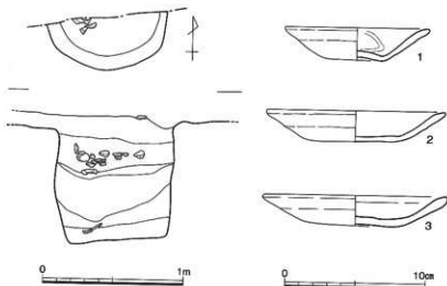
第367図 SK209実測図 (1/30)
