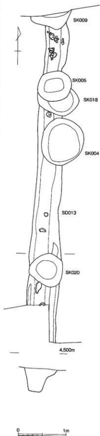
第415図 SD013実測図 (1/40)
