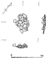
第387図 SX214実測図(1/30)
