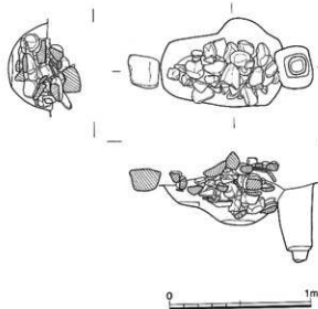
第383図 SX169 実測図 (1/30)
