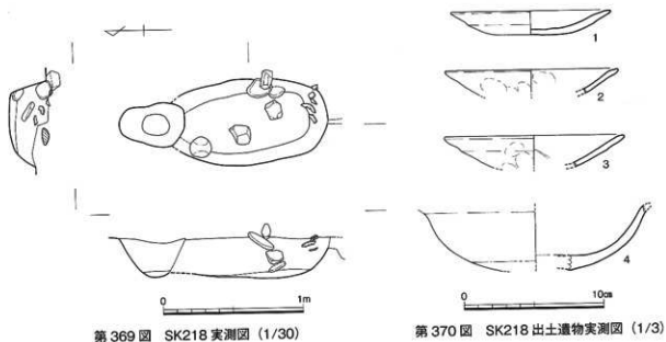
第369図 SK218 実測図 (1/30)
