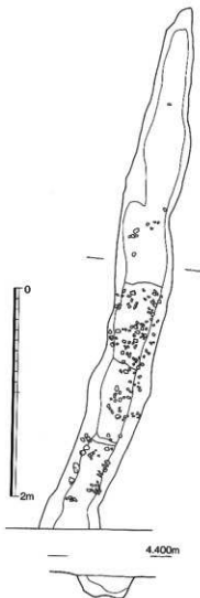
第426図 SD040 実測図 (1/40)
