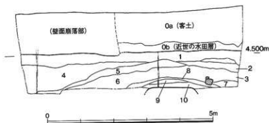
第352図 調査区東壁土層実測図 (1/80)
