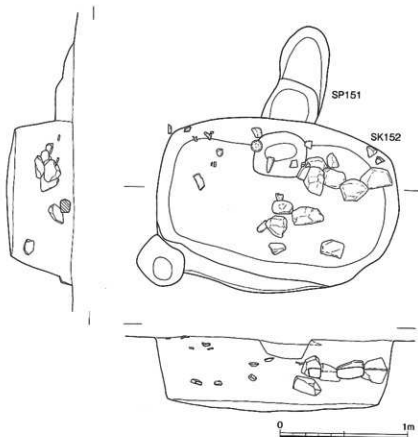
第353図 SK152 実測図 (1/30)
