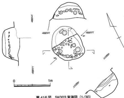
第416図 SK003実測図(1/30)
