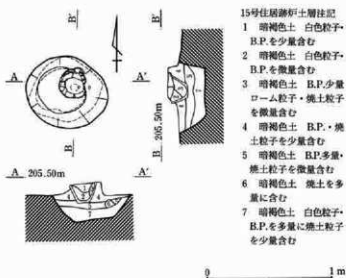
第22図 15号住居跡炉
