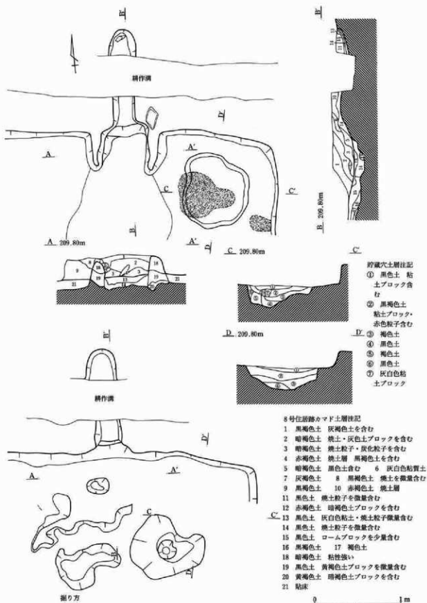
第297図 8号住居跡カマド
