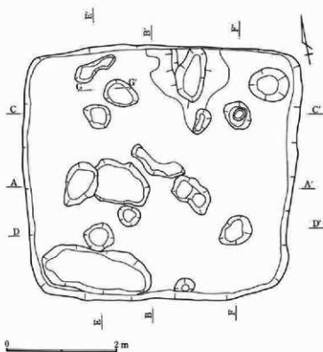
第304図 11号住居跡掘り方
