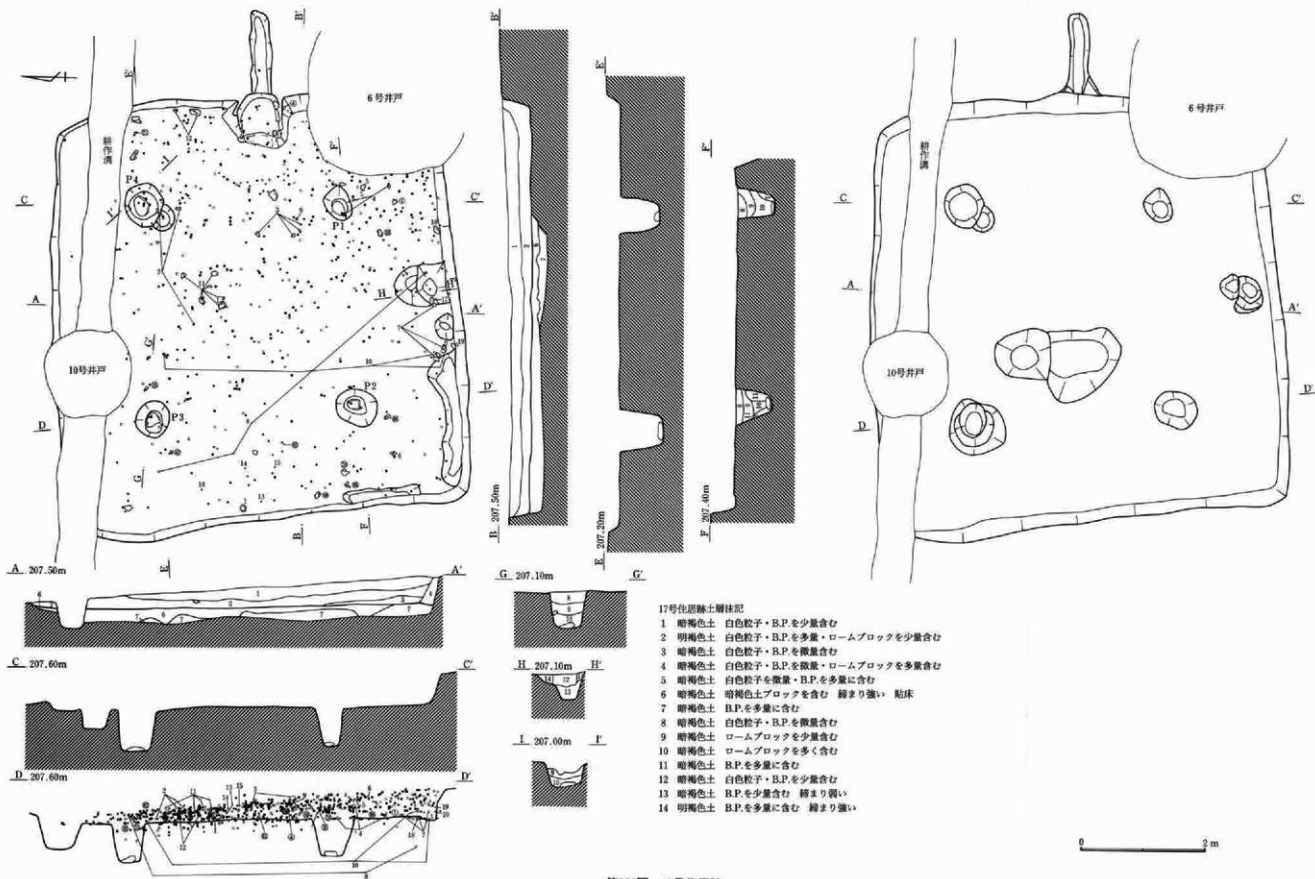
第322図 17号住居跡
