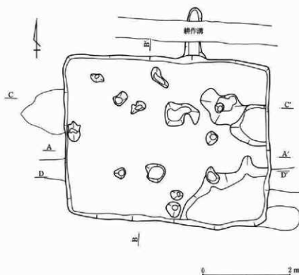
第295図 8号住居跡掘り方
