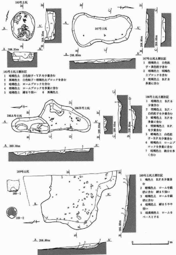
第67図 185～187・189号土坑
