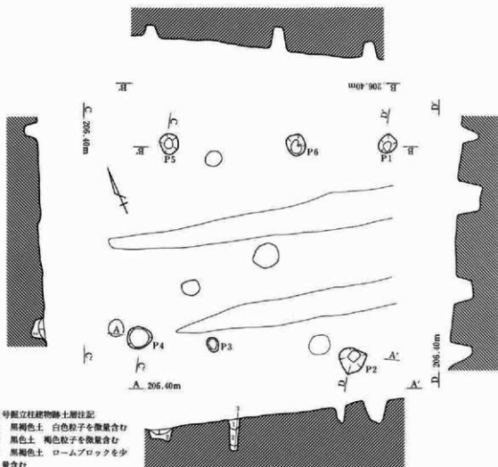
第381図 3号掘立柱建物
