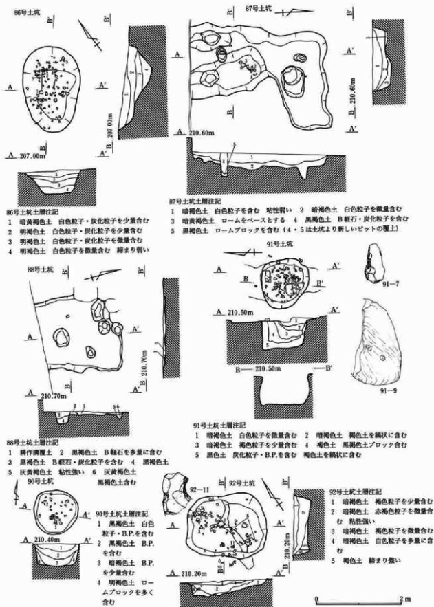
第56図 86～88・90～92号土坑
