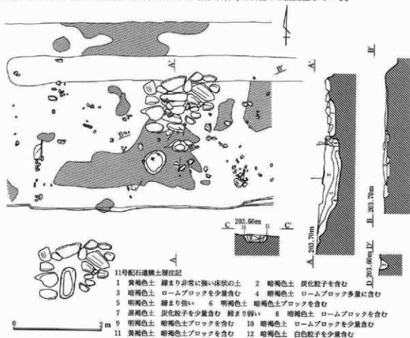
第374図 11号配石遺構
