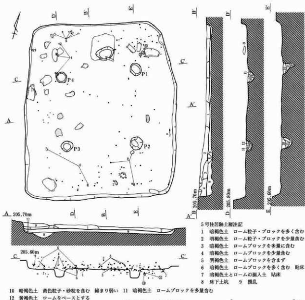
第257図 5号住居跡
