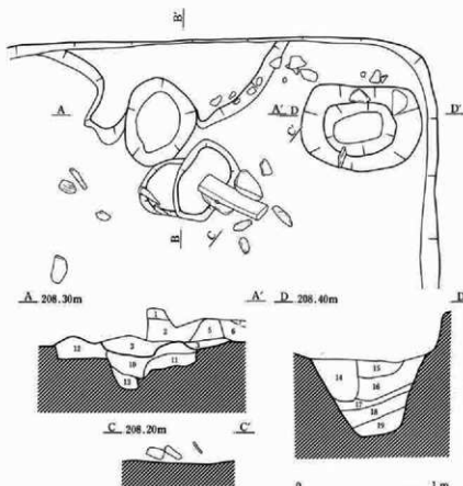
第305図 11号住居跡カマド
