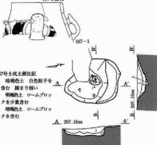
第64図 158・162~165・167号土坑
