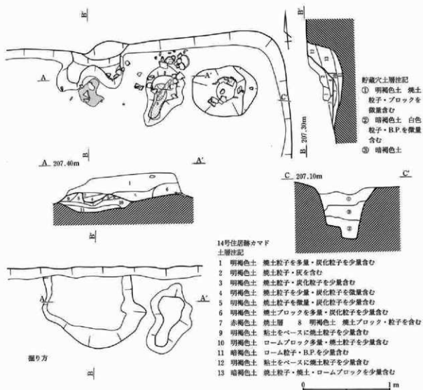
第319図 14号住居跡カマド
