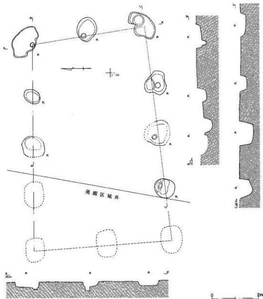
第480図 第5号掘立柱建物跡
