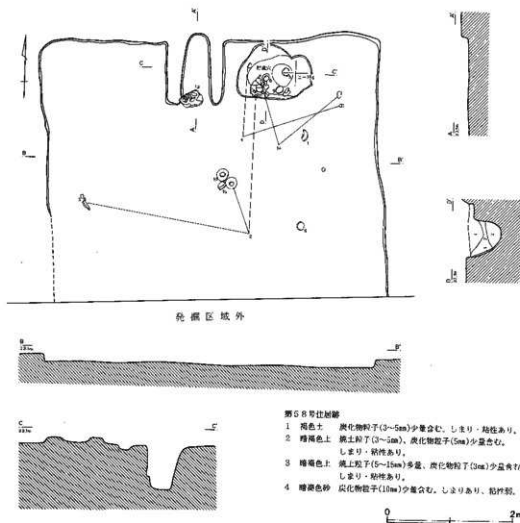
第350図 第58号住居跡
