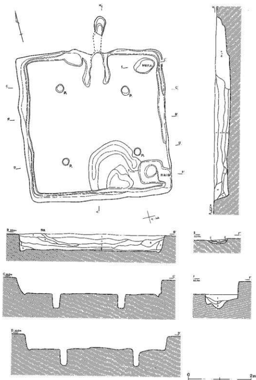
第187图 第15号住居跡(1)
