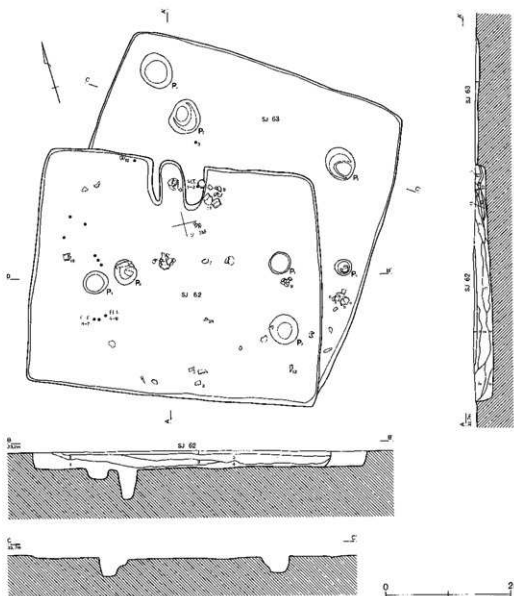
第62・63号住居跡
