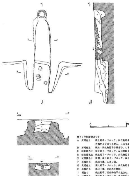
第300図 第47号住居跡(2)
