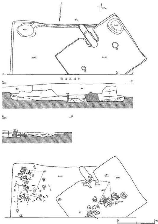
第278图 第41·42号住居跡(1)
