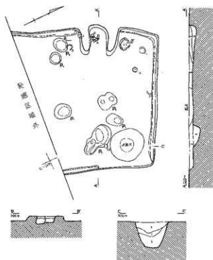
第456図 第91号住居跡
