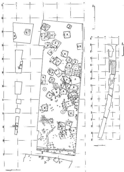
第322岡 第2発掘区全測図
