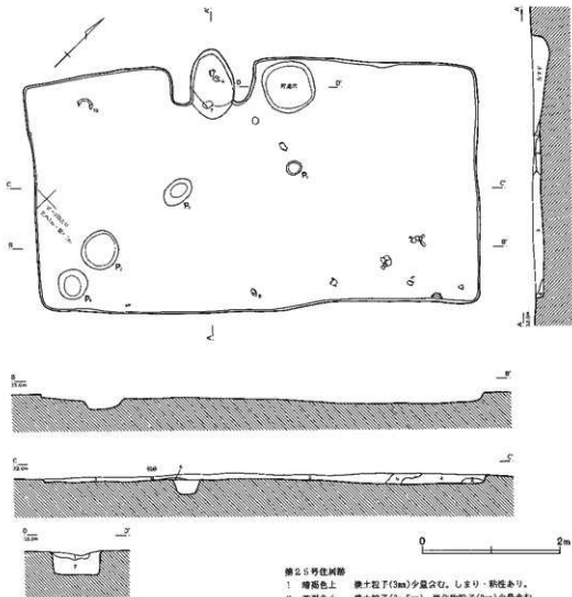
第25号住居跡野面図
