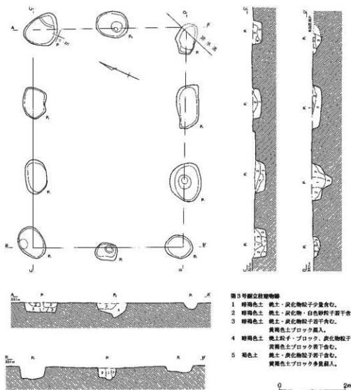
第478図 第3号竪立柱建物跡
