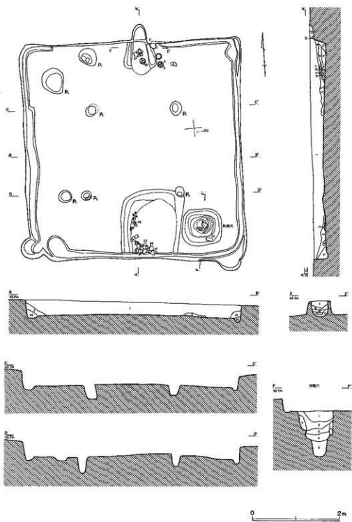
第450图 第88号住居跡
