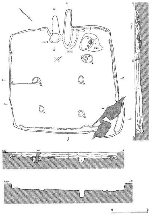
第396图 第71号住居跡(1)
