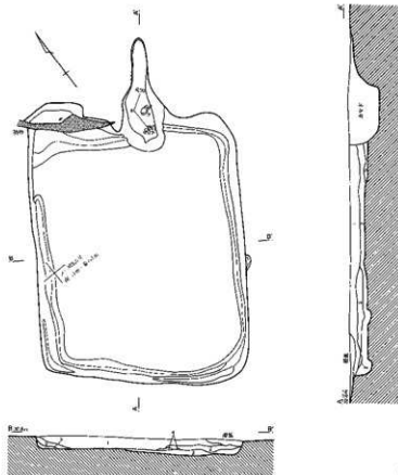
第141図 第4号住居跡(1)
