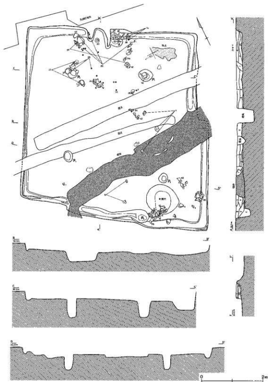
第345图 第57号住居跡(2)
