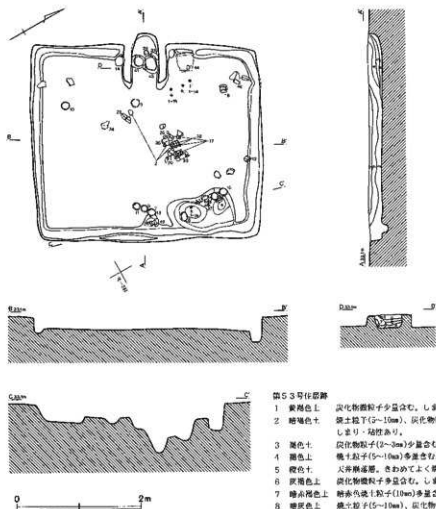
第331図 第53号住居跡
