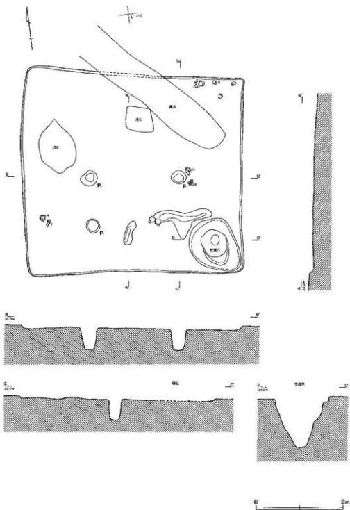
第324图 第50号住居跡
